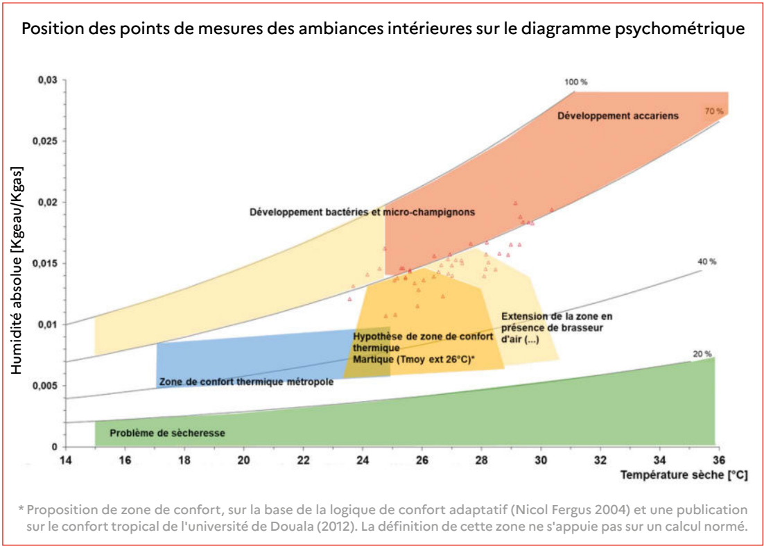
Répartition des points de mesure sur le diagramme psychrométrique
