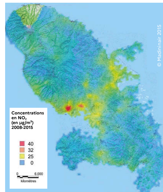
Cartographie des concentrations en dioxyde d'azote NO 2 (gaz traceur de la pollution automobile) en Martinique
