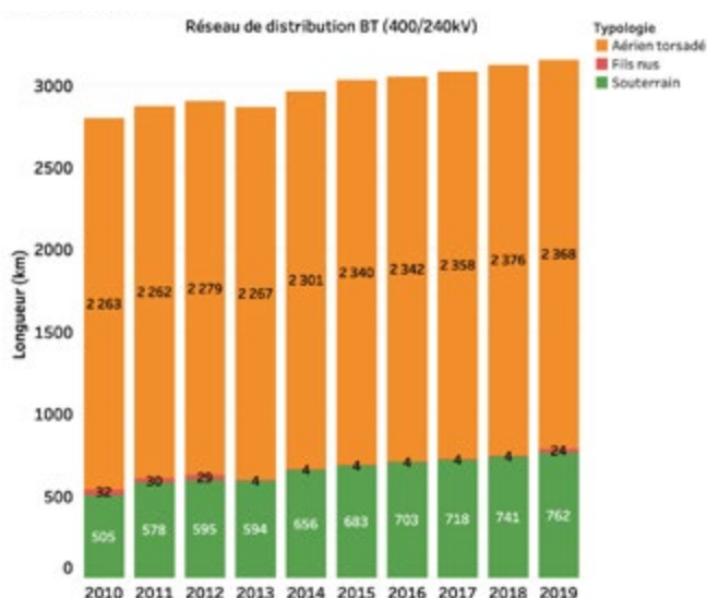
Figure 34: Evolution du réseau BT (Basse tension) de 2010 à 2019 (Données sources : EDF Martinique– Auteur : OTTEE)
