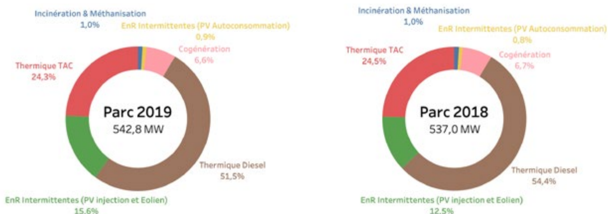
Figure 23 : Répartition du parc électrique en 2019 et 2018 par typologie (Données sources : EDF Martinique, Exploitants PV – Auteur : OTTEE)
