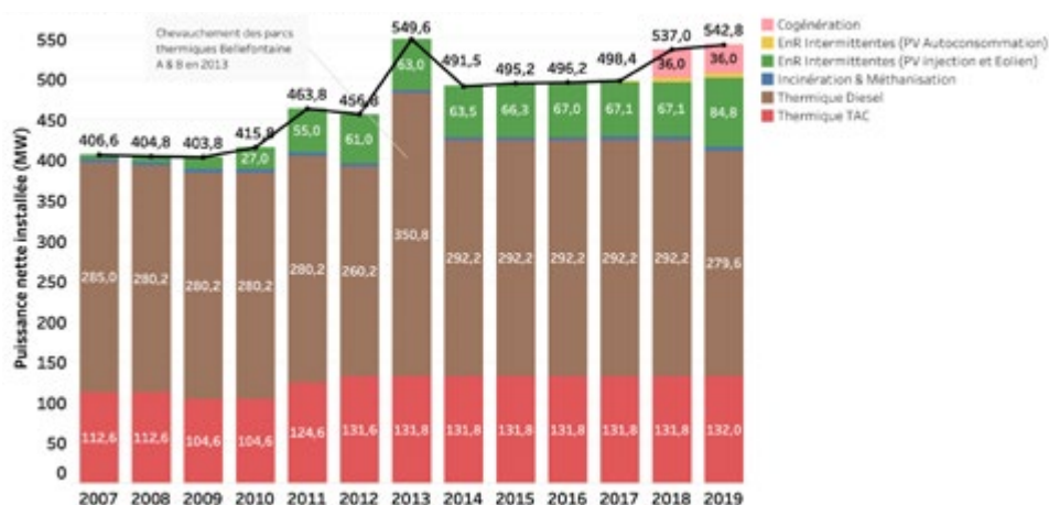
Figure 24 : Evolution du parc électrique de 2007 à 2019 par typologie
