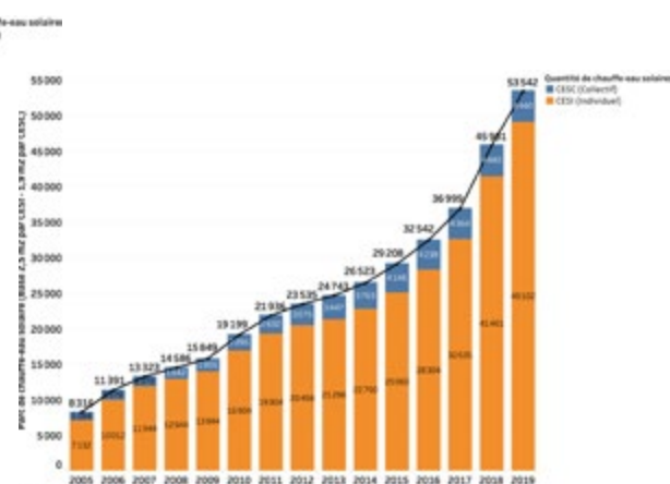
Figure 78 : Evolution du parc annuel de chauffe-eaux solaires de 2005 à 2019
