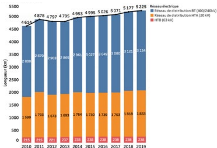
Figure 33 : Evolution du réseau électrique martiniquais de 2011 à 2019 par typologie (Donnée sources : EDF Martinique– Auteur : OTTEE)
