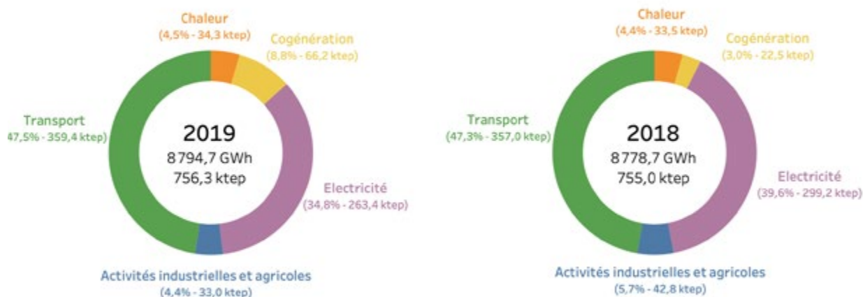
Figure 20 : Destination des ressources énergétiques primaires en 2018 et 2019 (Données sources : SARA/Grand Port Maritime/EDF/ADEME/Producteurs d'électricité/Obser'ver – Auteur : OTTEE)
