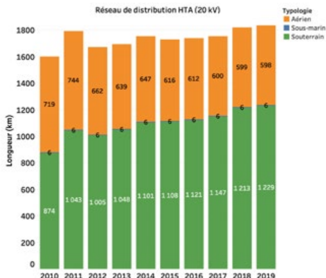
Figure 35: Evolution du réseau HTA (20 kV) de 2010 à 2019 (Données sources : EDF Martinique– Auteur : OTTEE)
