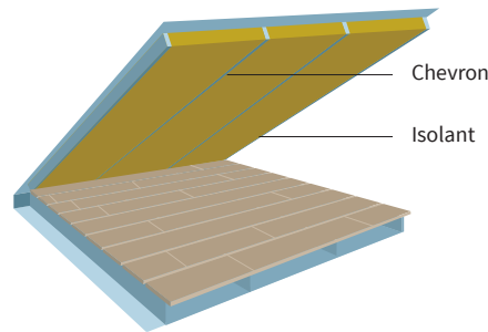
ISOLATION PAR L'EXTÉRIEUR
