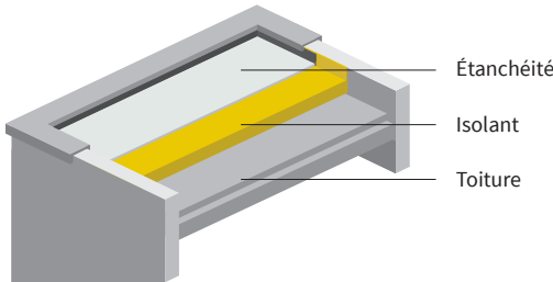
ISOLATION PAR L'EXTÉRIEUR
