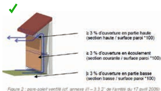
Figure 2 : pare-soleil ventilé (cf. annexe II – 3.3.2 de l'arrêté du 17 avril 2009)
