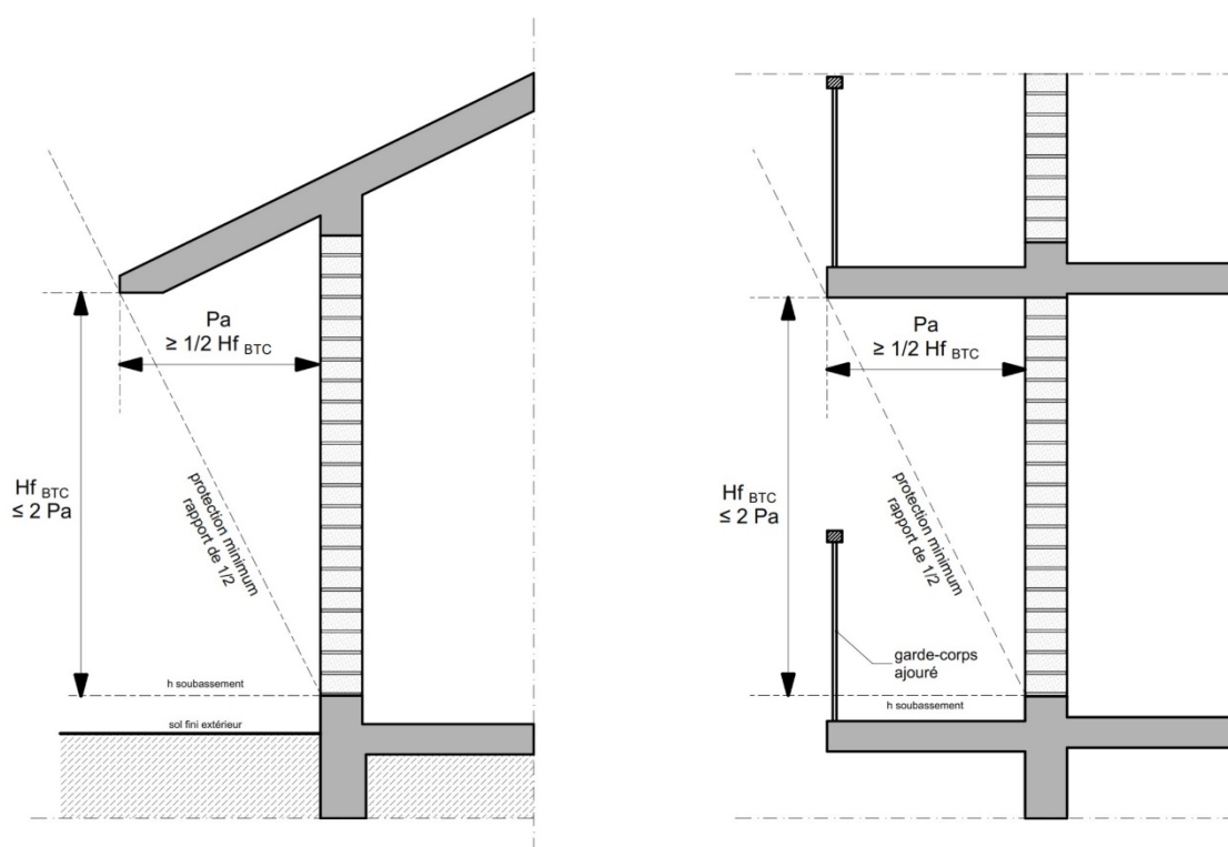
FIGURE 7 : FAÇADE ABITÉE, PRINCIPE SCHEMATIQUE DE LA PROFONDEUR DE L'ABRI – DÉBORD DE TOITURE, BALCON ET LOGGIA
