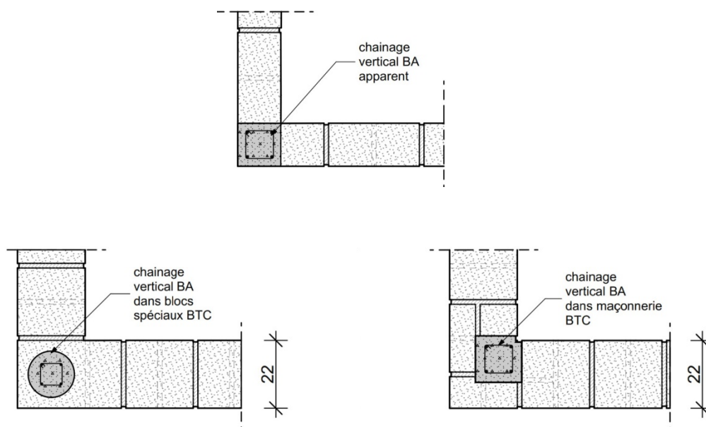
FIGURE 48 : PRINCIPES DE CHAÎNAGES VERTICAUX EN BETON ARME
