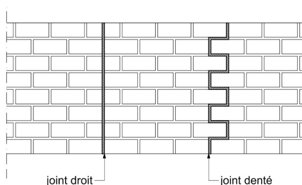
FIGURE 27 : JOINTS DE RETRAIT, DISPOSITIONS DE PRINCIPES, VUES EN ÉLEVATION
