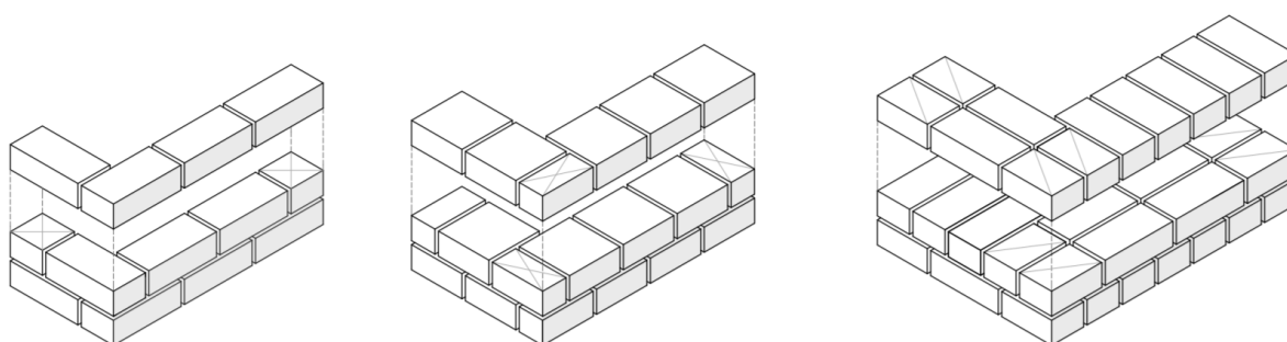
FIGURE 17 : ANGLES DE MUR SIMPLE ET DOUBLE ÉPAISSEUR DE BTC – épaisseurs 14, 22, 29,5 cm
