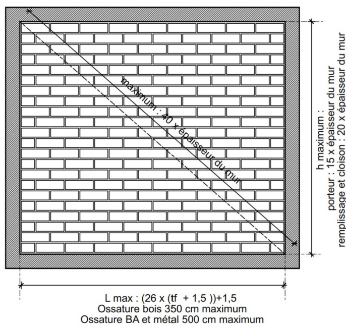
FIGURE 10 : DIMENSIONS MAXIMALES : LONGUEUR, HAUTEUR ET DIAGONALE DES PANNEAUX DE MAÇONNERIE
