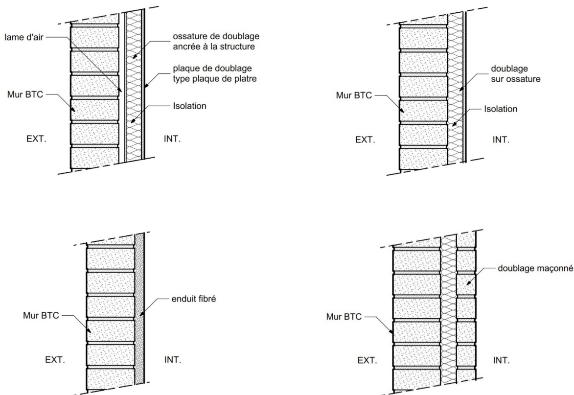
FIGURE 43 : COUPE DE PRINCIPE DES DOUBLAGES ISOLANTS (ITI)
