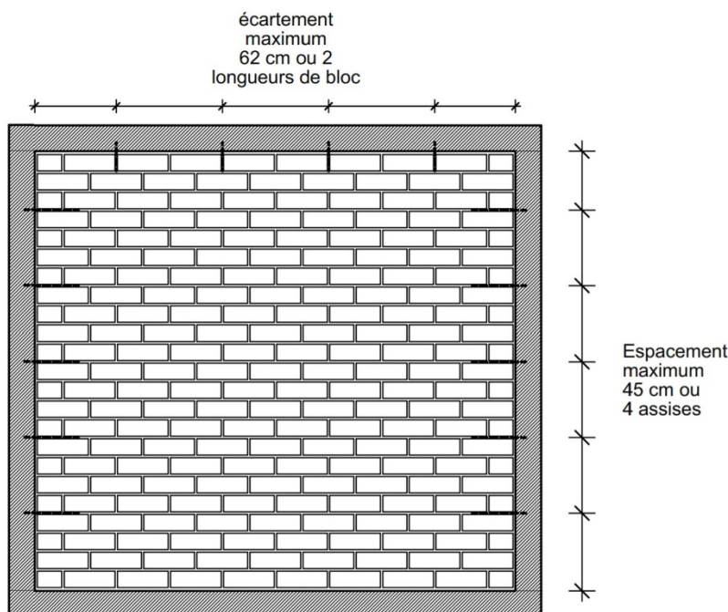
FIGURE 62 : ÉLEVATION DE PRINCIPE DE LA RÉPARTITION DES ATTACHES DE LIAISON DANS LES DEUX DIRECTIONS
