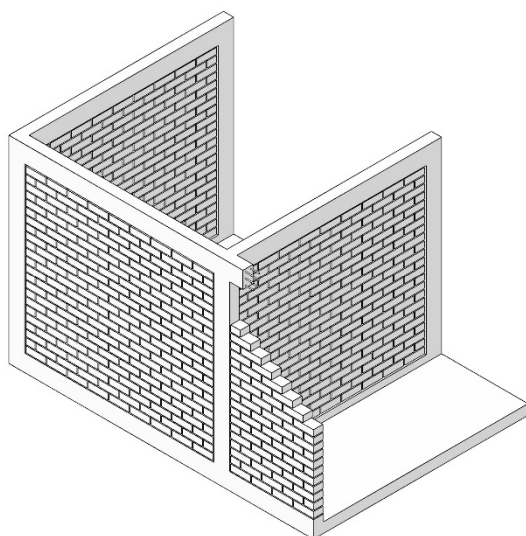
c. Remplissage d'ossature métal
