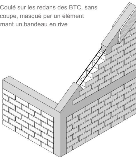
FIGURE 49 : PRINCIPES DE CHAÎNAGE INCLINÉ EN BETON ARMÉ
