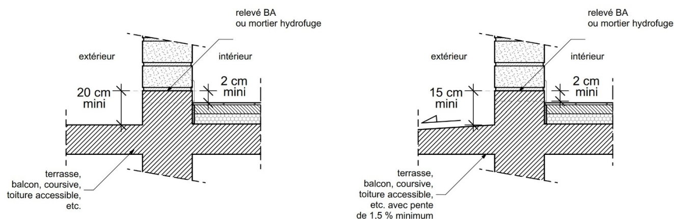
FIGURE 23 : COUPES DE PRINCIPE — PIED DE MUR SUR BALCON, TERRASSE, ETC.
