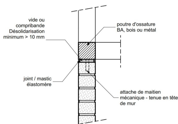
FIGURE 57 : COUPE DE PRINCIPLE SCHÉMATIQUE - OSSATURE BÉTON, BOIS OU MÉTAL / LIAISONS EN TÊTE DE MUR PAR ATTACHES PONCTUELLES
