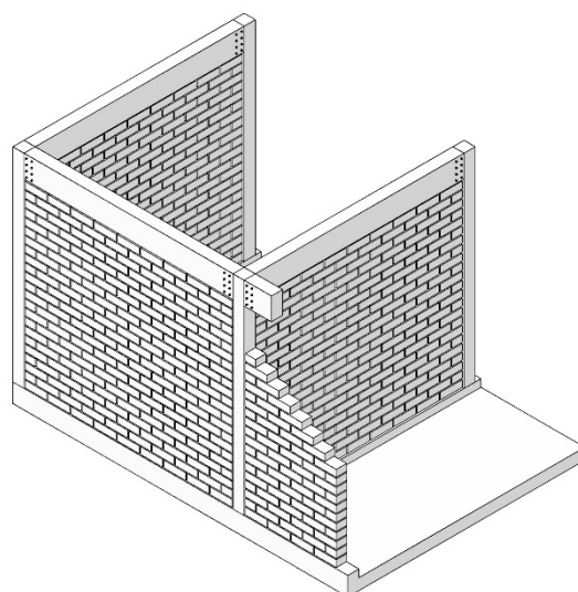
b. Remplissage d'ossature bois
