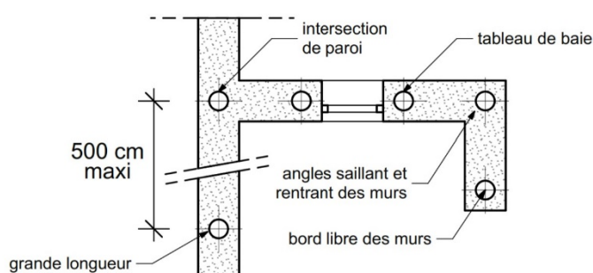
FIGURE 47 : PLAN DE PRINCIPES DES CHAÎNAGES VERTICAUX
