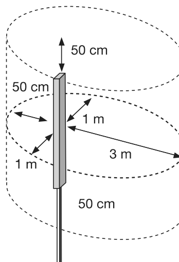
Figure 9.12 : exemple de zone d'installation interdite autour d'une antenne émettrice de téléphonie mobile
