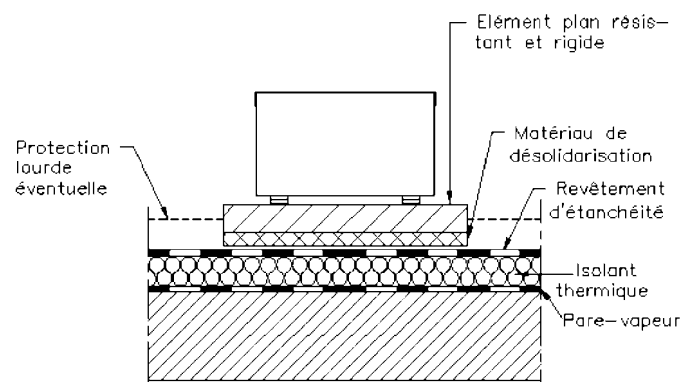
Figure 9.14 : exemple de mise en œuvre caisson
