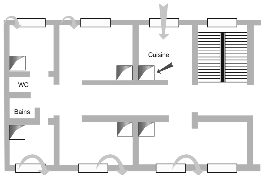
Figure 3.2 : aération par ouvrants
