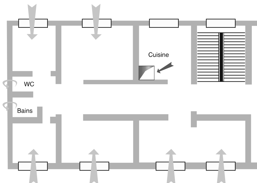
Figure 3.4 : ventilation partielle
