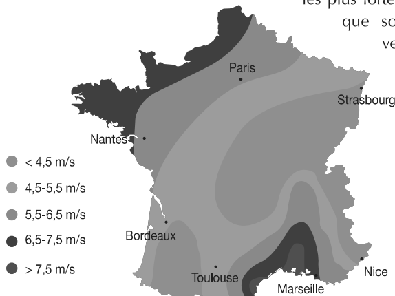
Figure 4.3 : ressource éolienne à 50 m
