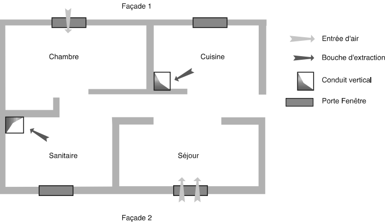
Figure 8.3 : schéma d'implantation
