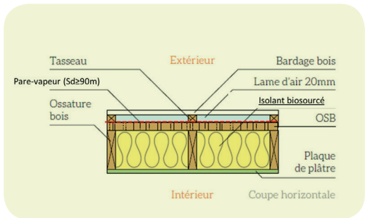
Figure 26 : Exemple de mur à ossature bois – Cas particulier d'un bâtiment climatisé à une altitude inférieure à 400 m
