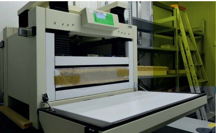
La mesure de conductivité thermique (en W \cdot m^{-1} \cdot K^{-1} ) des prototypes a été réalisée au lambdamètre selon la norme NF EN 12667 (2001) sur des échantillons de 600 mm x 600 mm x 100 mm (figure 8)
