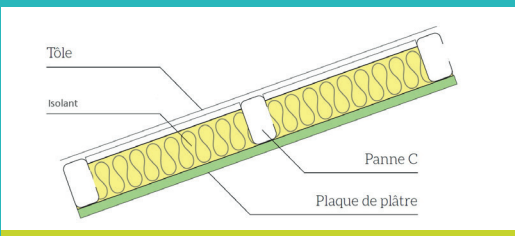
Figure 9. Types de parois verticales et horizontales sélectionnées
