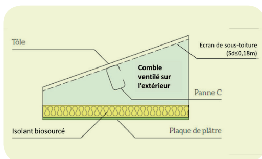
Figure 23 : Exemple de comble perdu – Cas général
