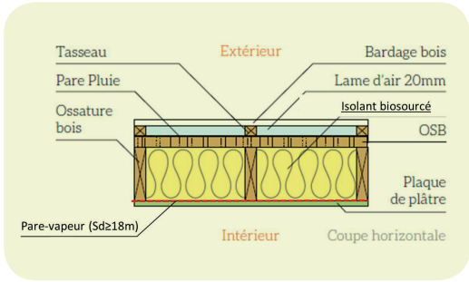
Figure 27 : Exemple de mur à ossature bois – Cas particulier d'un bâtiment à une altitude supérieure à 800 m
