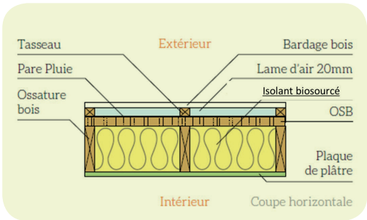
Figure 25 : Exemple de mur à ossature bois – Cas général
