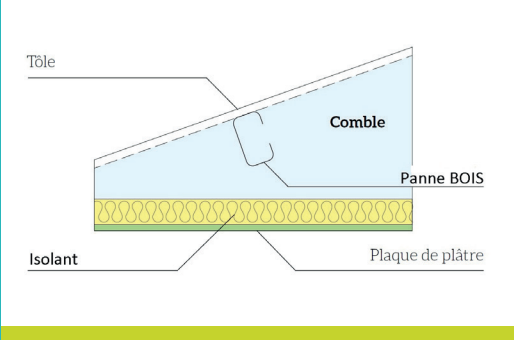
Figure 9. Types de parois verticales et horizontales sélectionnées
