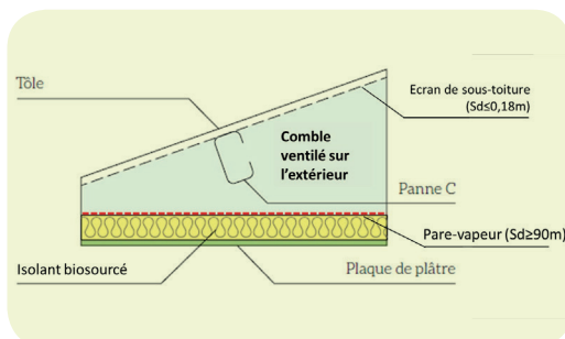
Figure 24 : Exemple de comble perdu – Cas particulier d'un bâtiment climatisé à une altitude inférieure à 400 m
