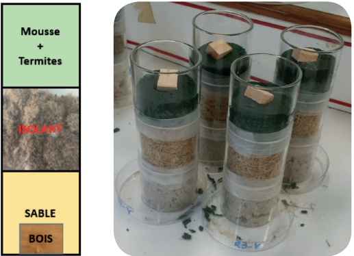
Figure 19. Dispositifs d'essais réalisés selon la norme XP X 41550 adaptée
