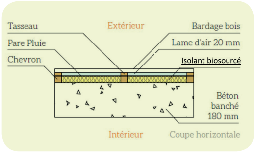
Figure 28 : Exemple de parois en maçonnerie ou béton isolées par l'extérieur
