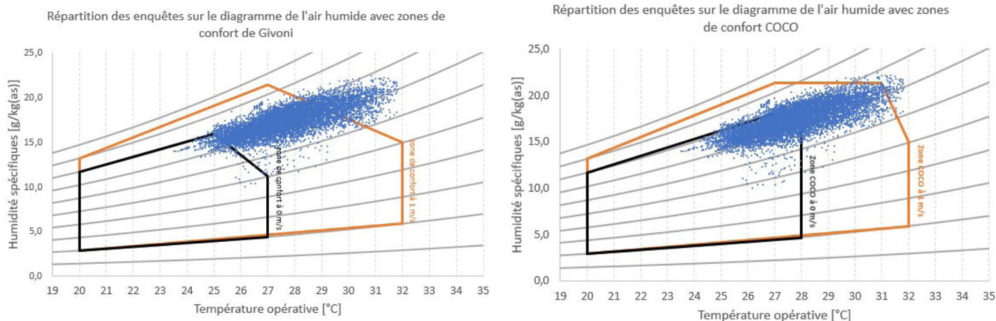
Figure 13 : Comparatif du diagramme de Givoni (à gauche) et de COCO (à droite) pour un logement
