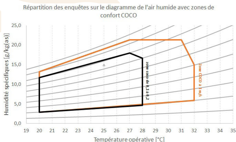
Figure 12 : Diagramme de confort COCO 5
