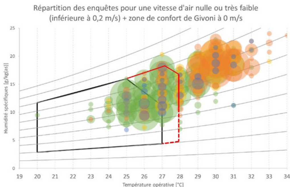
Figure 9 : proposition d'agrandissement de la zone de confort à vitesse d'air nulle à très faible en rouge
