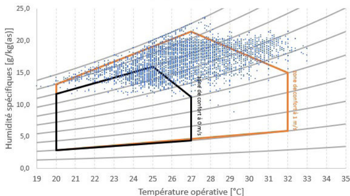
Répartition des enquêtes sur le diagramme de l'air humide avec zones de confort de Givoni
