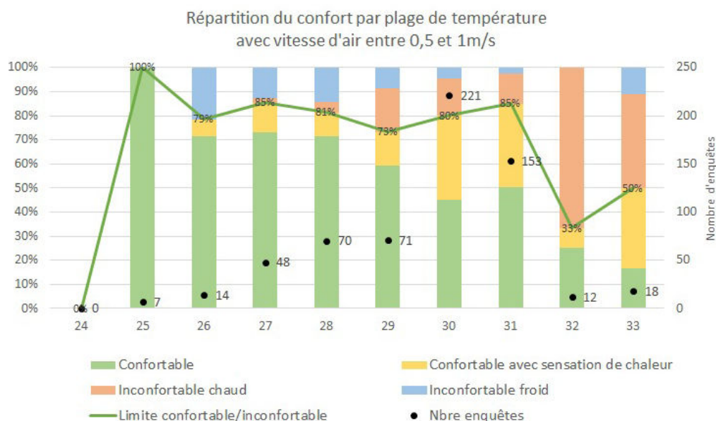
Figure 10 : répartition du confort par plage de température pour une vitesse d'air entre 0,5 et 1 m/s – 646 enquêtes sur les 2 territoires
