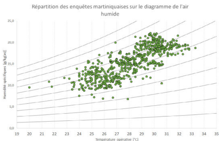
Figure 4 : La répartition des enquêtes martiniquaises sur le diagramme de l'air humide
