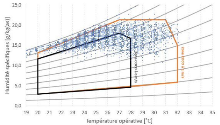
Répartition des enquêtes sur le diagramme de l'air humide avec zones de confort COCO
