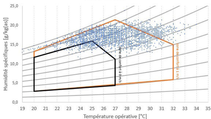
Répartition des enquêtes sur le diagramme de l'air humide avec zones de confort de Givoni
