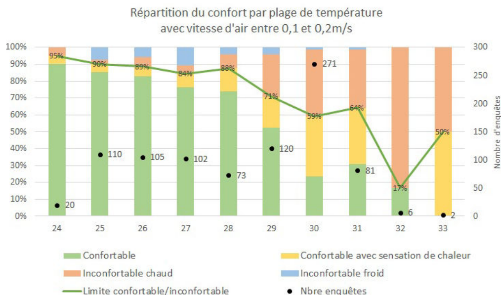
Figure 8 : répartition du confort par plage de température pour les enquêtes avec une vitesse d'air nulle à très faible – 1 701 enquêtes sur les 2 territoires
