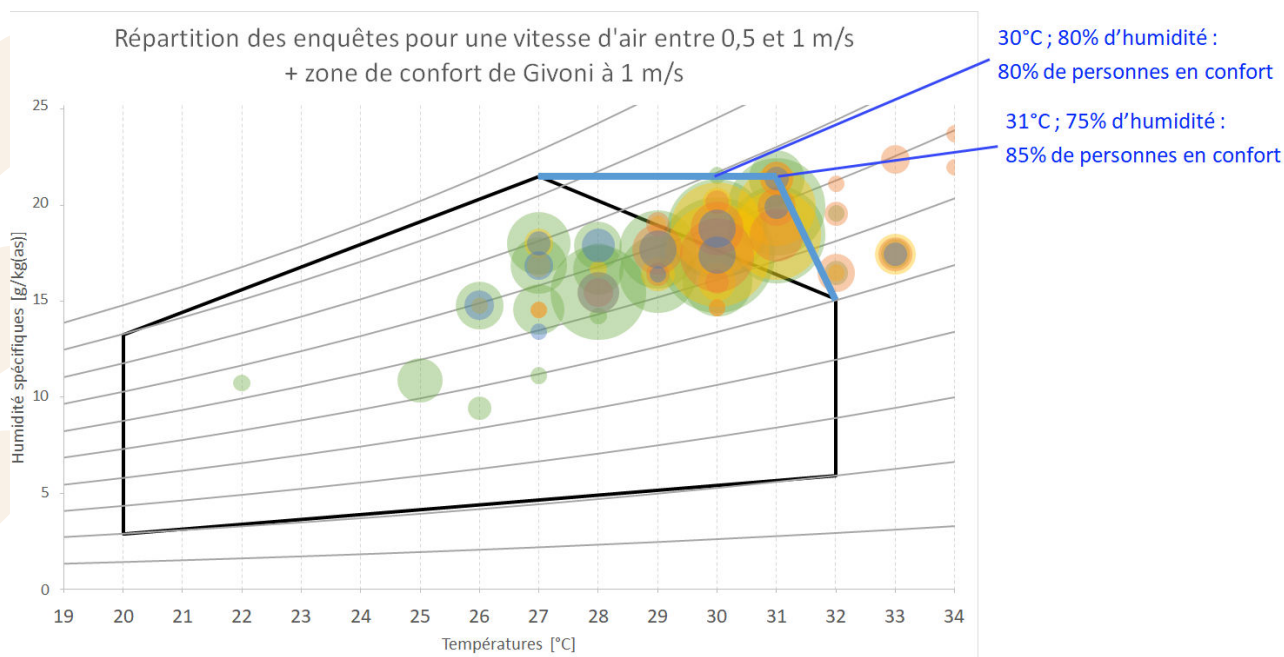
Figure 11 : proposition d'agrandissement de la zone de confort à 1 m/s en bleu
