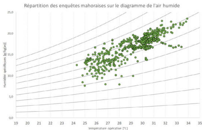
Figure 5 : La répartition des enquêtes mahoraises sur le diagramme de l'air humide
