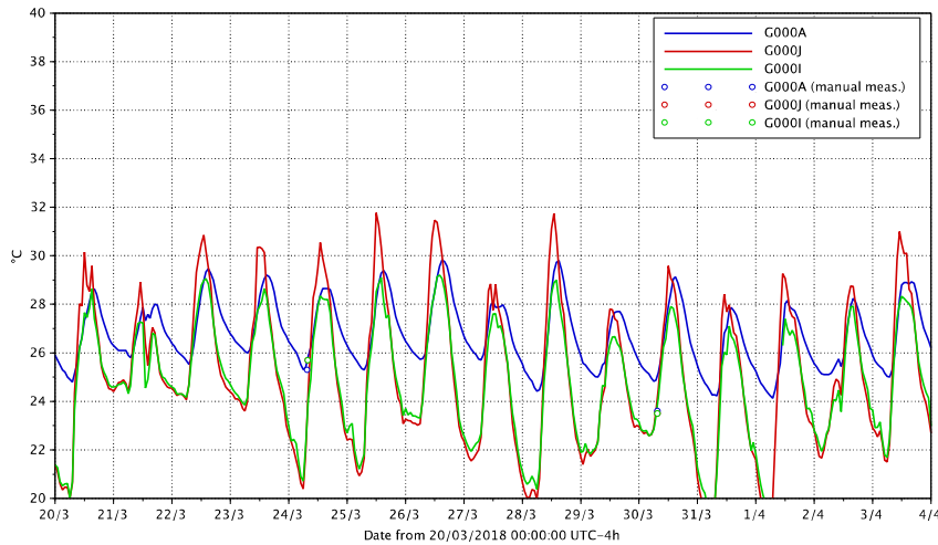
Figure 25 : Mesure des températures de l'air sur le site G000
