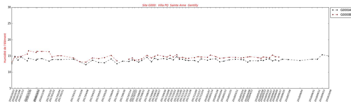
Figure 32 : Evolution humidité du bois en fonction du temps Site G000 éléments intérieurs abrités Résineux
