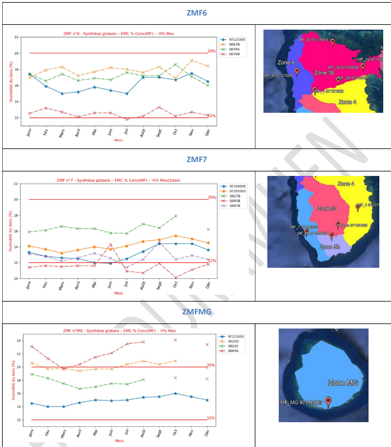
Figure 47 : Courbes Humidité mesurée du Bois résineux abrités extérieurs par ZMF -Guadeloupe
