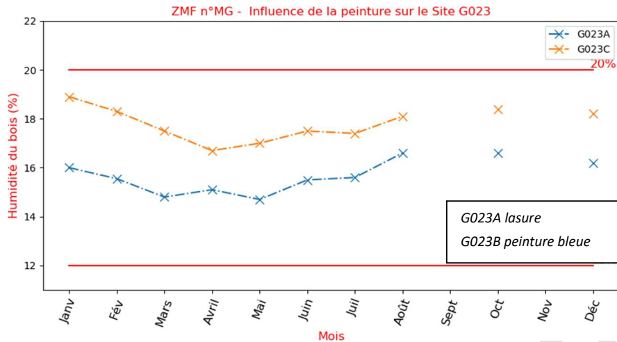
Figure 71 - Évolution de l'humidité de deux poteaux au revêtement différent du site G023 en fonction du temps
