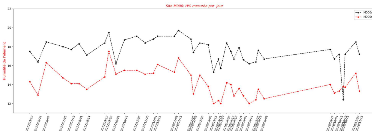
Figure 33 : Evolution humidité du bois en fonction du temps Site M000 éléments extérieurs abrités
