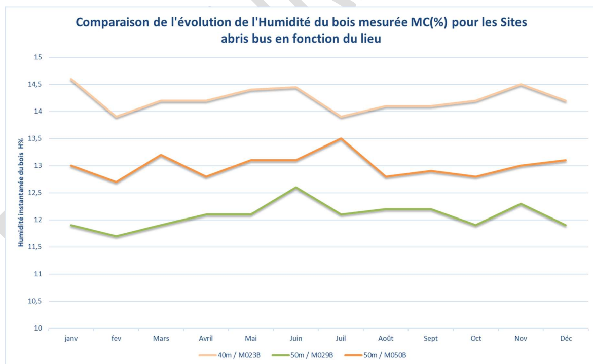
Figure 57 : Graphes d'humidité des Sites type « Abri bus Angelim Vermelho Martinique
