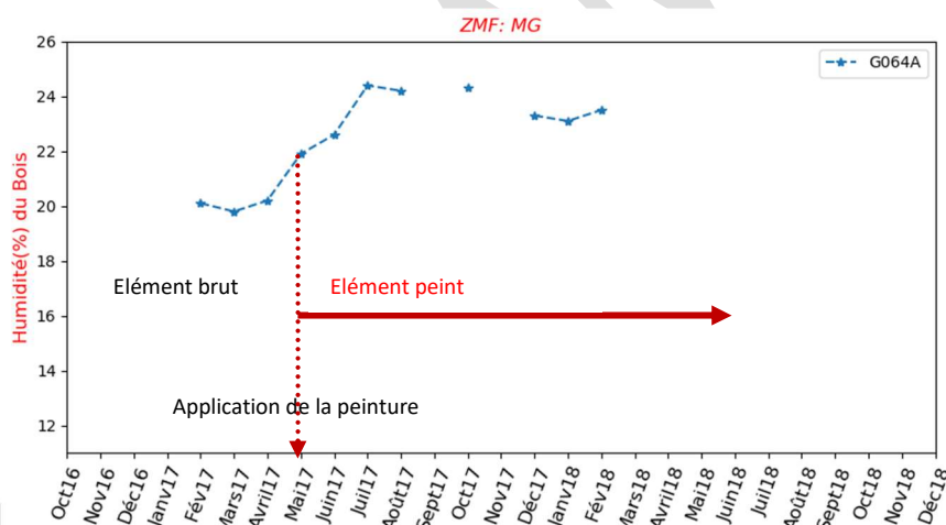
Figure 73 - Évolution de l'humidité d'une poutre après application d'un revêtement - Site G064
