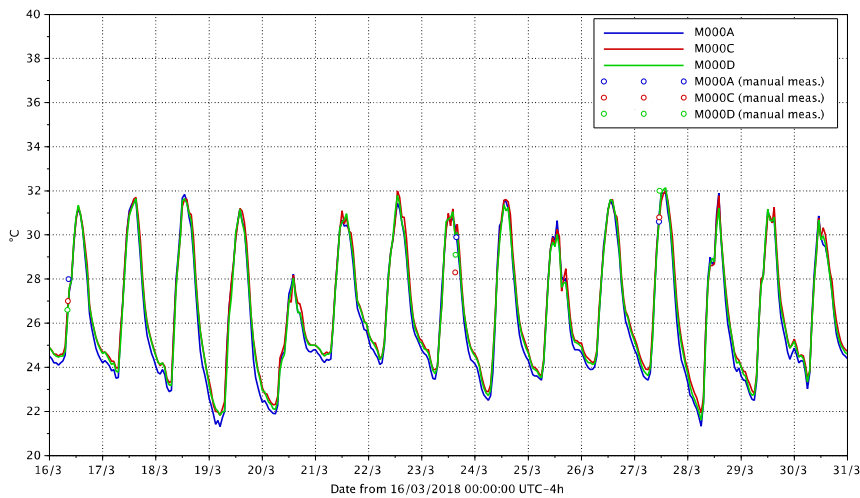
Figure 26 : Mesure des températures de l'air sur le site M000
