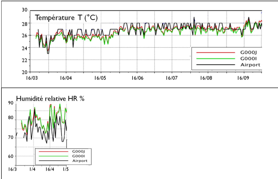
Figure 30 : Comparaison mesures monitoring/Données MF
