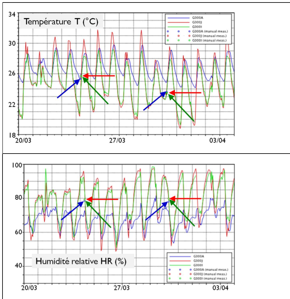
Figure 31 : Comparaison mesures monitoring/mesures sites
