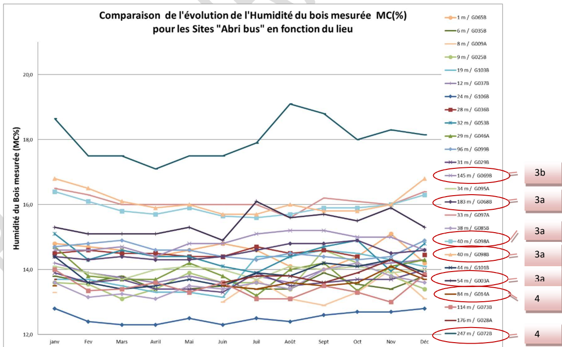
Figure 55 : Graphes d'humidité des Sites type « Abri bus Angelim Vermelho »- Guadeloupe
