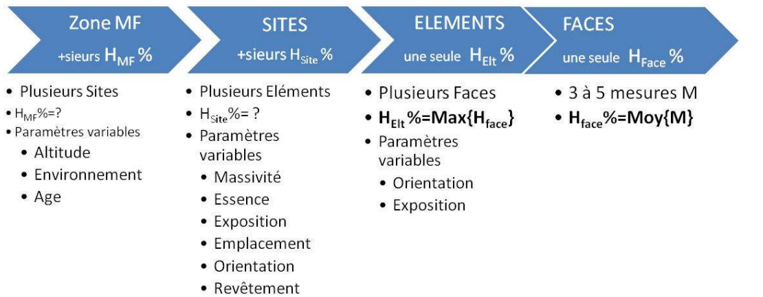
Figure 13 : Humidité du bois et paramètres considérés suivant les différentes échelles d'observation
