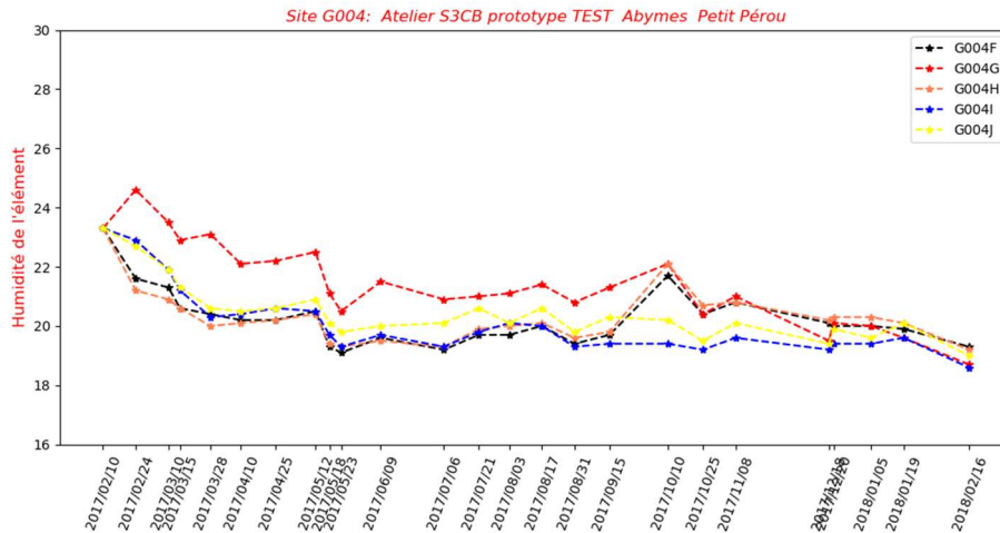
Figure 74 - Évolution de l'humidité des 5 échantillons non peints en fonction du temps
