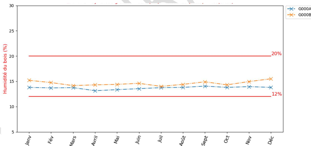
Figure 44 : Exemple de variation des mesures moyennées sur 1 an pour 2 Eléments
