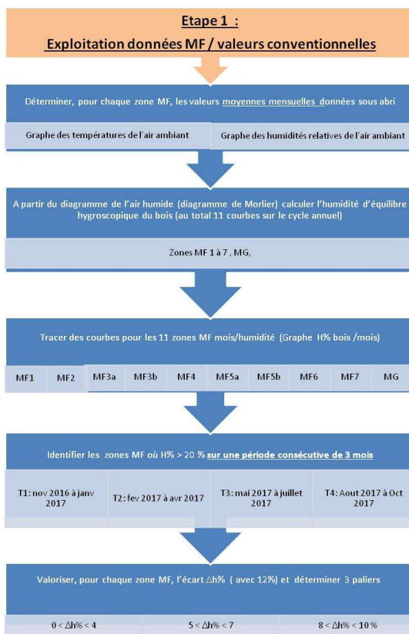
Figure 35 : Démarche de l'étape 1 BOIS-DURAMHEN
