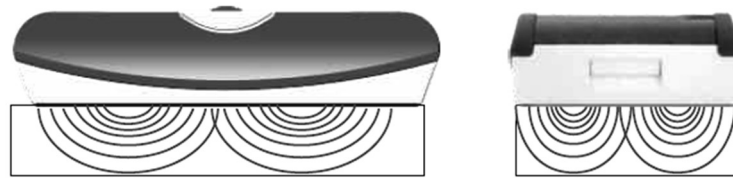
Figure 9 : Champ d'émission de l'humidimètre nécessitant une hauteur et largeur suffisantes [Merlin]
