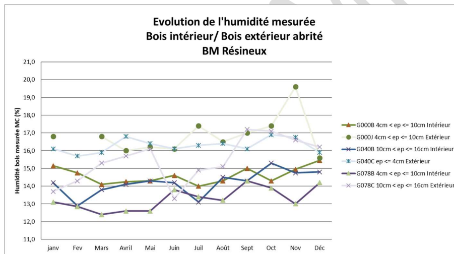
Figure 62 : Comparaison humidité des Eléments intérieurs et extérieurs au sein d'un même Site
