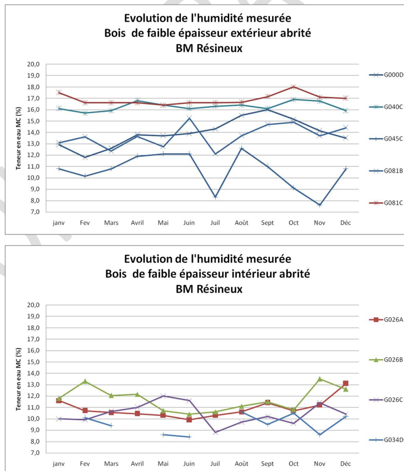
Figure 78 : Graphes d'humidité des Bois influence de la massivité - Guadeloupe
