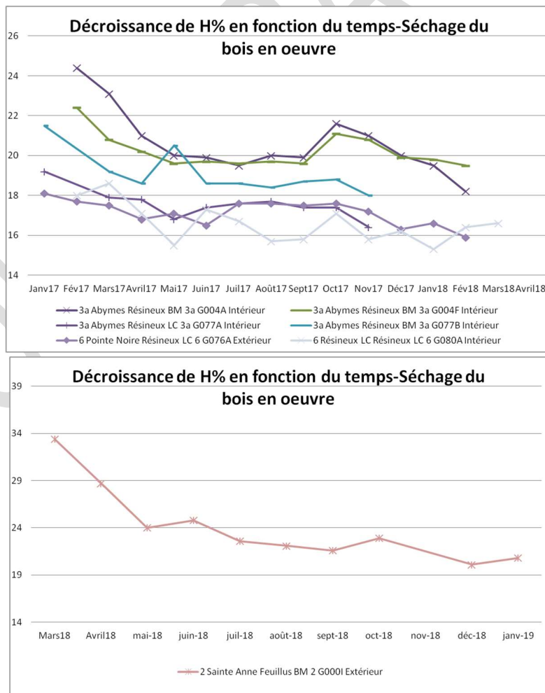
Figure 65 : Graphes d'humidité des Bois mis en œuvre avant séchage
