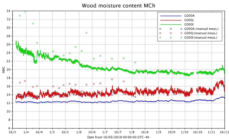
Figure 23 : Mesures de H% sur les pièces du site G000
