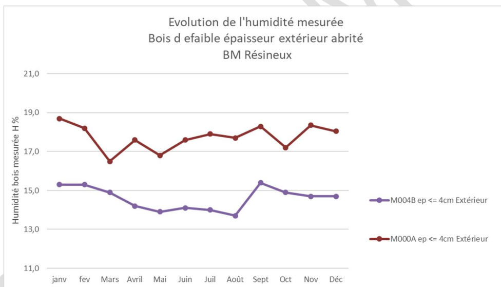
Figure 80 : Graphes d'humidité des Bois influence de la massivité BM Résineux -Martinique
