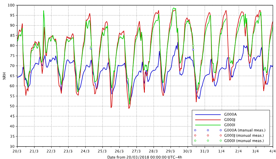
Figure 27 : Mesure des humidités relatives de l'air sur le site G000
