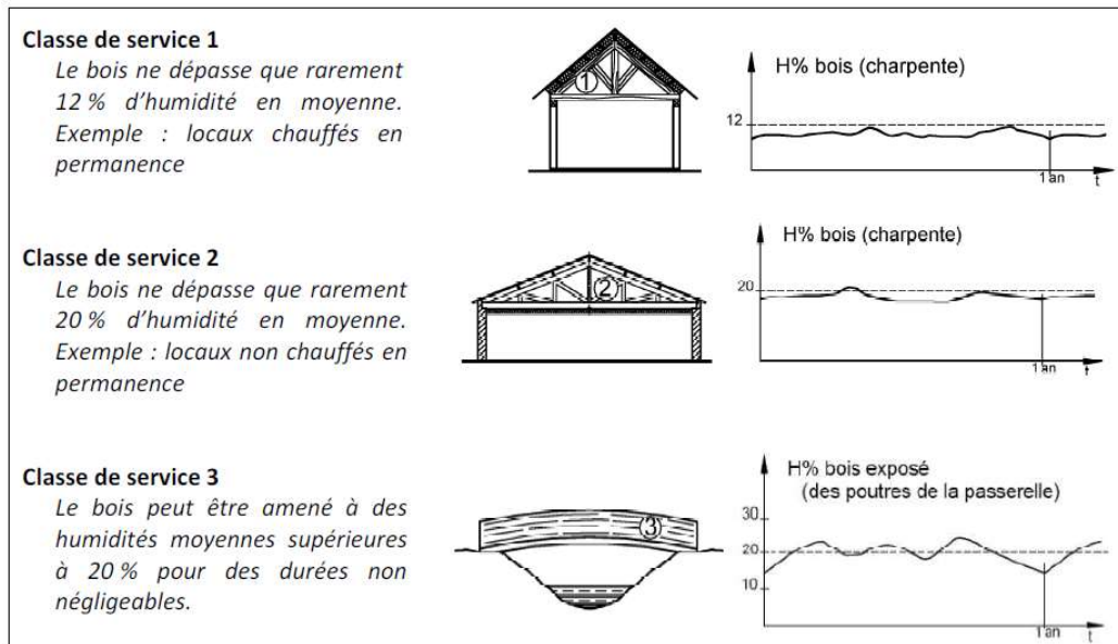
Figure 1 : Classes de service et exemples d'application
