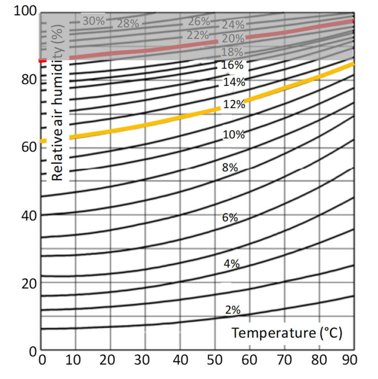
Figure 22 : Utilisation possible du diagramme d'équilibre hydrique des bois de l'EN 1995-1.1/NA
