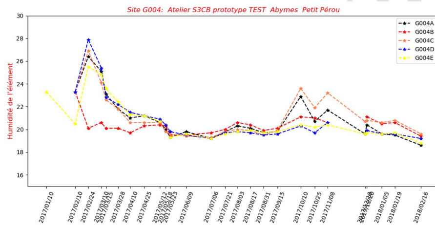
Figure 75 - Évolution de l'humidité des 5 échantillons peints en fonction du temps
