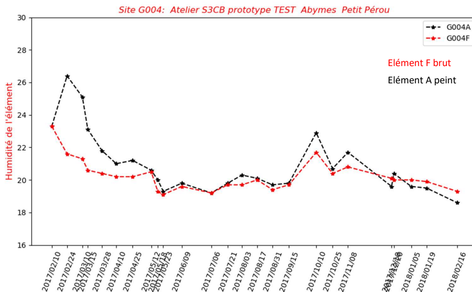
Figure 76 - Comparaison échantillons médians peint et non peint en fonction du temps
