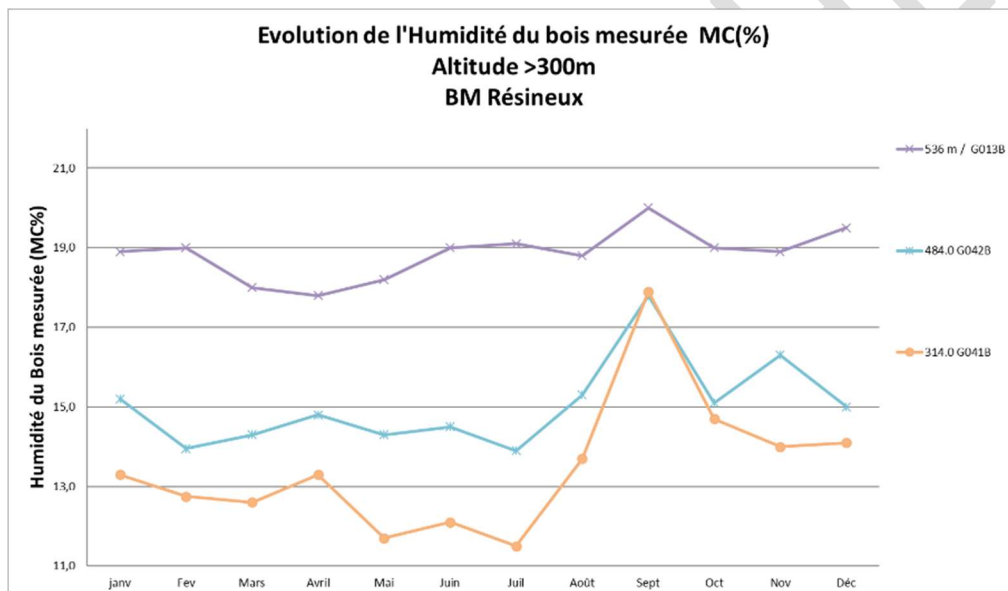
Figure 59 : Graphes d'humidité des Sites à une Altitude > 300m Guadeloupe
