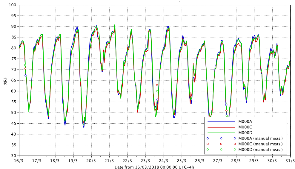
Figure 28 : Mesure des humidités relatives de l'air sur le site M000
