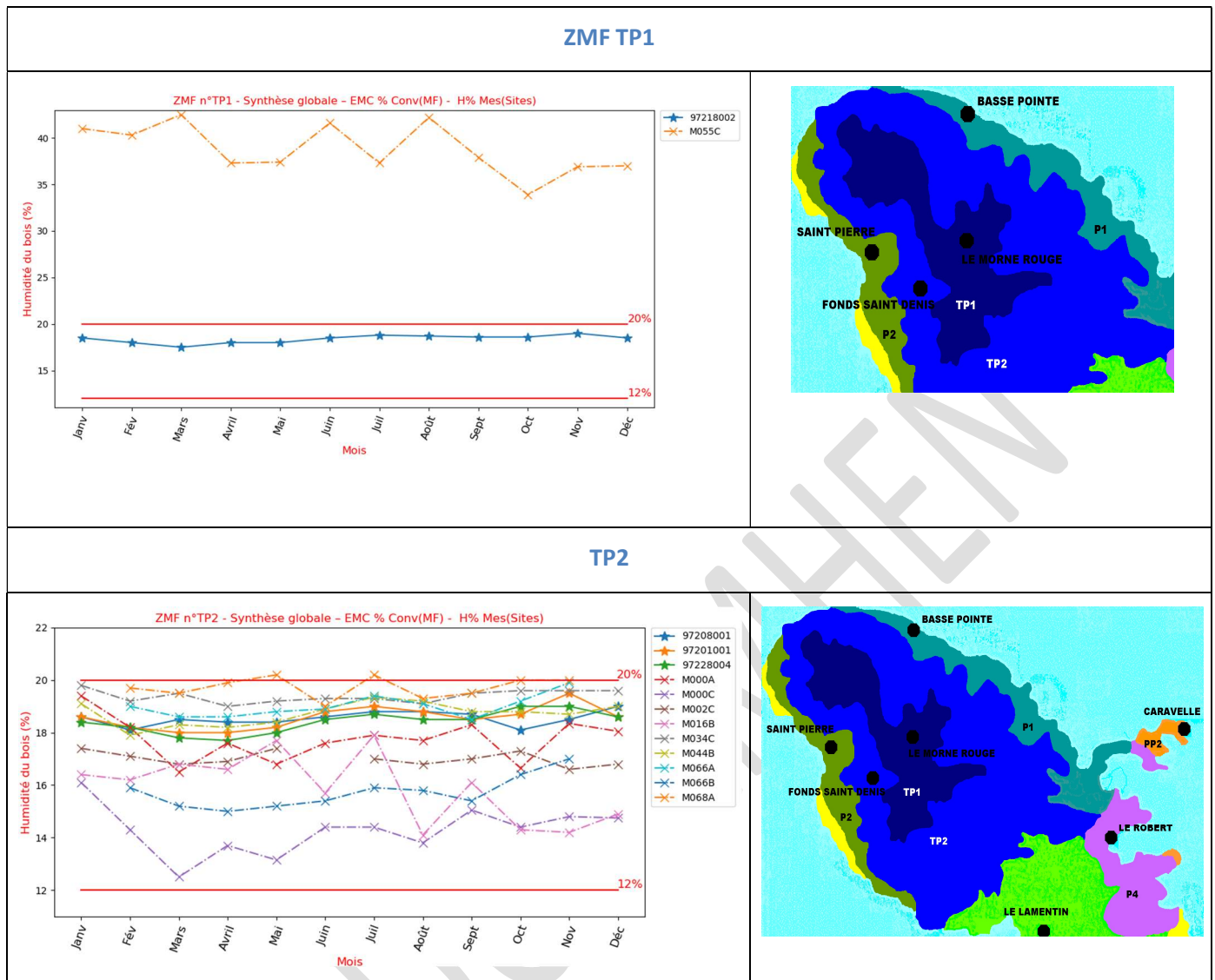
Figure 48 : Courbes Humidité mesurée du Bois résineux abrités extérieurs par ZMF -Martinique
