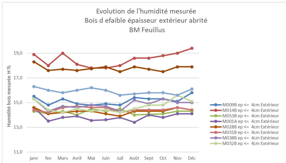
Figure 79 : Graphes d'humidité des Bois influence de la massivité BM Feuillus -Martinique
