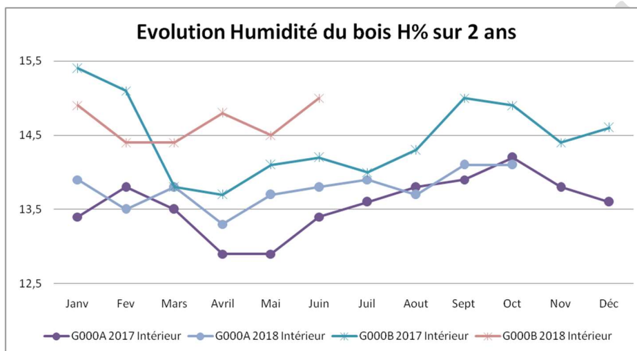
Figure 43 : Exemple de variation des mesures pour 2 Eléments sur 2 ans
