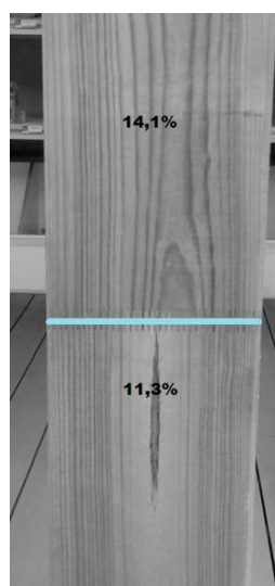
Figure 83 - Poteau abouté, mesures d'humidité moyennes du bois suivant les différents aboutages de la seconde face
