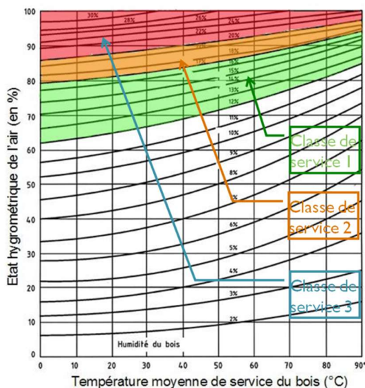
Figure 34 : Courbe d'équilibre hygroscopique définissant les classes de service
