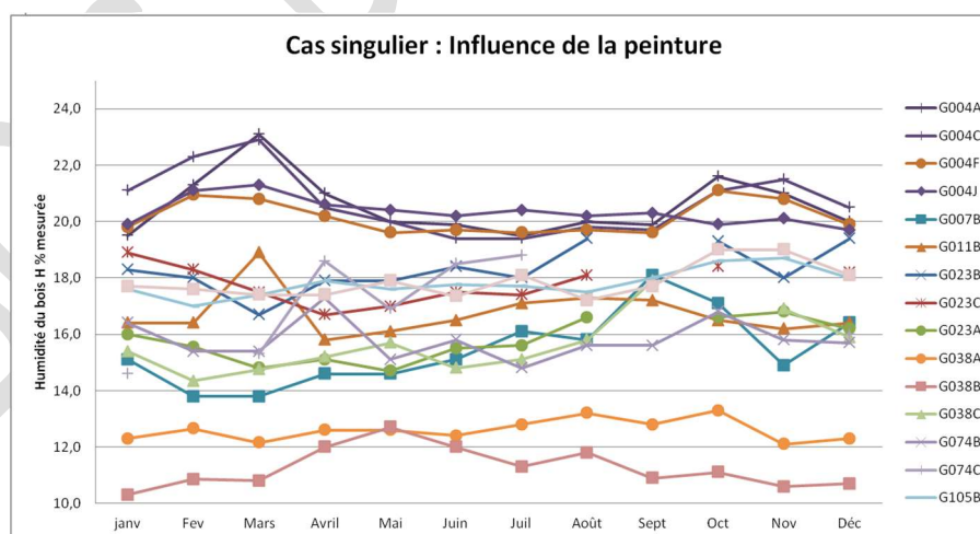
Figure 70 : Graphes d'humidité des Bois influence de la peinture Guadeloupe
