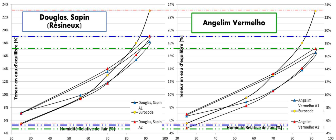
Figure 21 : Comparaison entre résultats obtenu et données issues de la courbe d'équilibre hydrique de la NF EN 1995-1.1/NA
