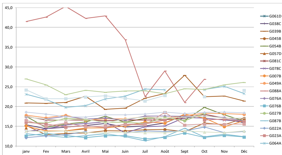
Figure 67 : Graphes d'humidité des Bois influence maritime Guadeloupe
