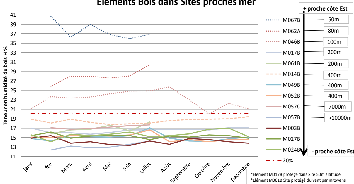
Figure 68 : Graphes d'humidité des Bois influence maritime -Martinique
