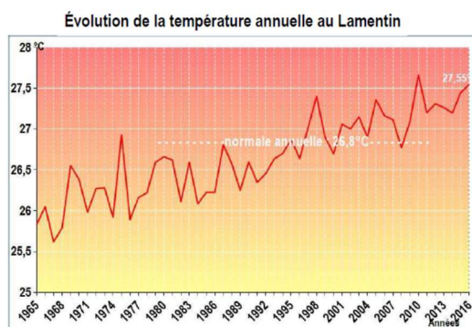
Figure 6 : Evolution de la température moyenne annuelle au Lamentin [7]
