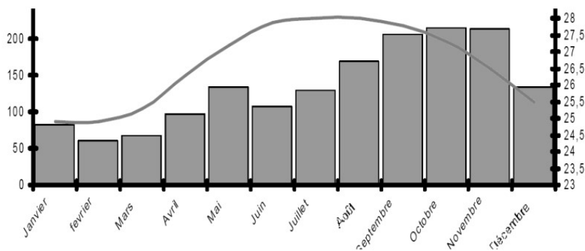
Figure 5 : Diagramme ombrothermique (températures et pluie) à Les Abymes Le Raizet[7]
