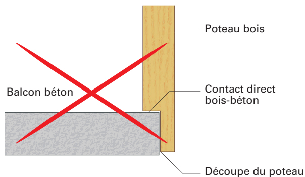
Figure 7 : Mauvaise conception d'un pied de poteau : appui partiel et contact direct avec le sol
