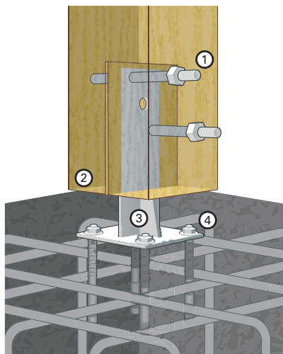
Figure 8 : Poteau en bois sur pied de poteau
