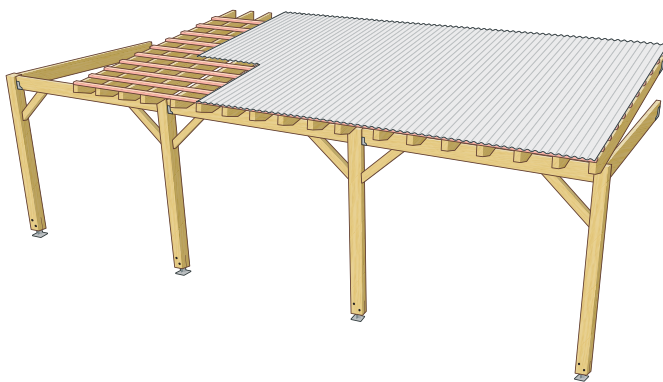
Figure 2 : Exemple d'auvent
