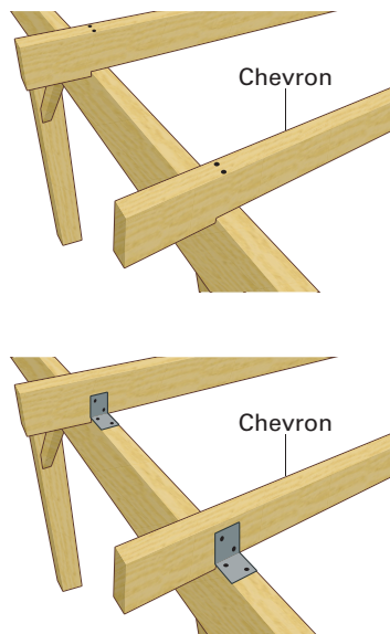
Figure 4 : Assemblage de toiture
