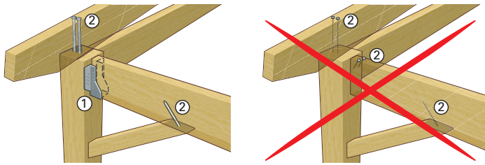
Figure 3 : Assemblages de toiture
