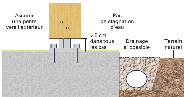
Figure 10 : Configuration possible en pied de poteau
