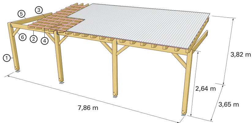
Figure 14 : Fixation de l'ouvrage au gros œuvre
