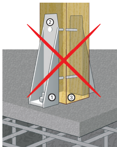
Figure 9 : Poteau en bois simplement appuyé au sol
