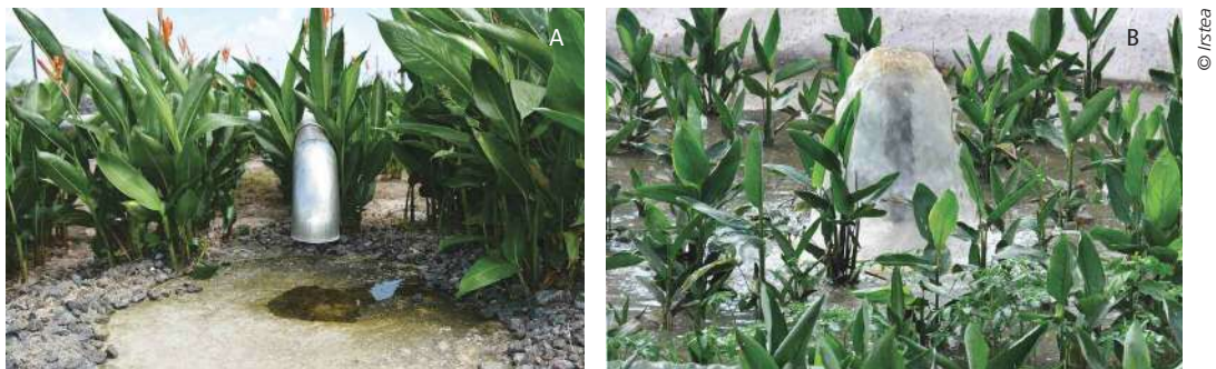
Figure 21. Réseau d'alimentation aérien avec la plaque anti-affoulement (à gauche), ou enterré lors d'une bâchée (à droite).
