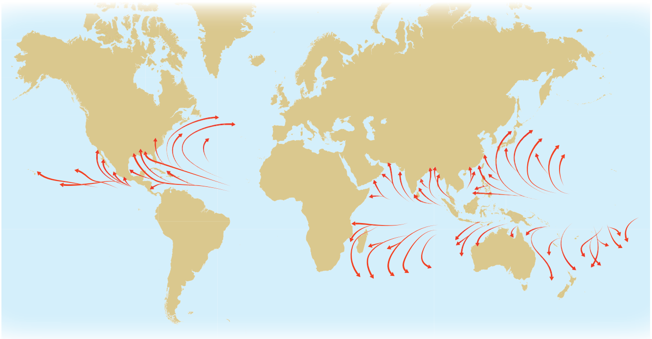
Figure 8 : Régions cycloniques
