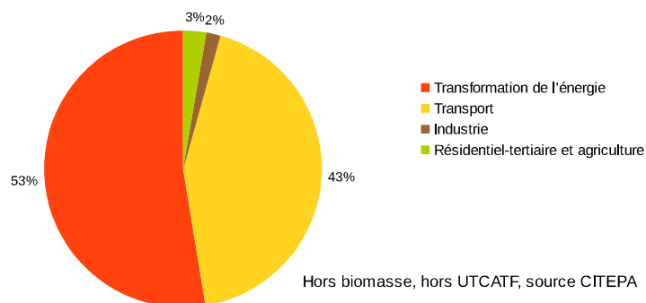
Répartition sectorielle des émissions de CO 2 en Martinique en 2015
