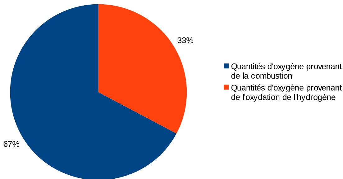
Oxygène nécessaire aux processus de combustion en Martinique
