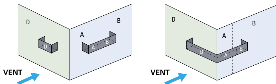
Figure 5 : Découpage des surfaces verticales du balcon ou de la coursive en fonction des zones de la façade
