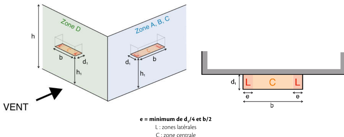
Figure 7 : Zones latérales et centrales de la surface horizontale du balcon ou de la coursive
