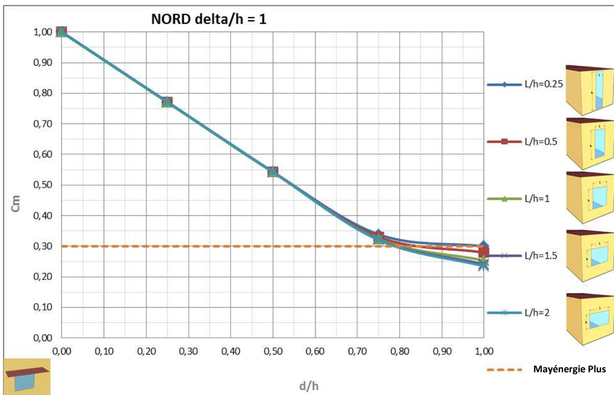
Figure 6-29 : Valeurs de C_m en fonction de la profondeur du débord pour une extension de débord \delta/h = 1 , pour des fenêtres orientées Nord
