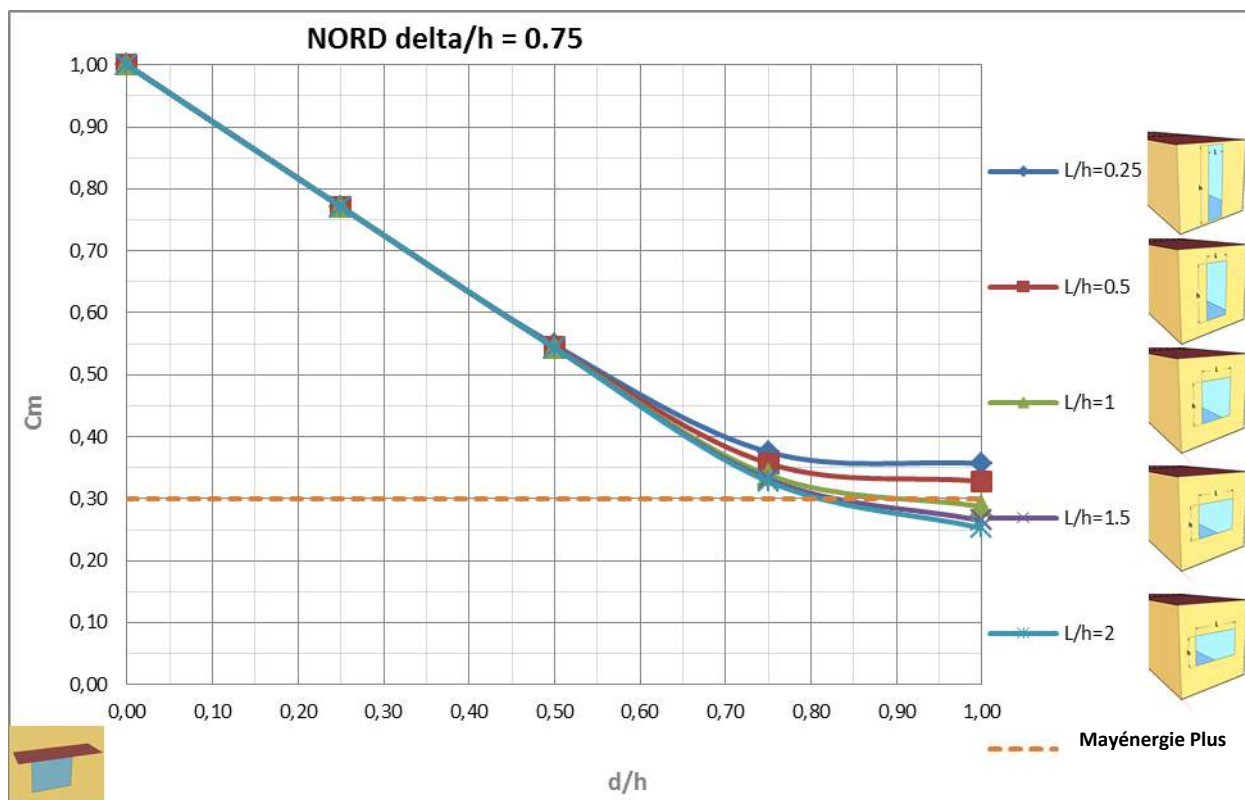
Figure 6-28 : Valeurs de C_m en fonction de la profondeur du débord pour une extension de débord \delta/h = 0.75 , pour différentes fenêtres orientées Nord
