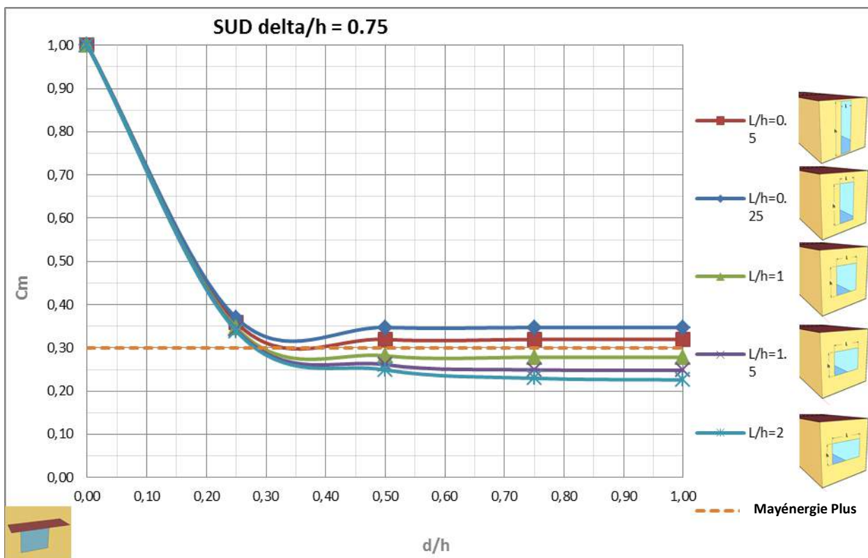
Figure 6-32 : Valeurs de C_m en fonction de la profondeur du débord pour une extension de débord \delta/h = 0.75 , pour des fenêtres orientées Sud
