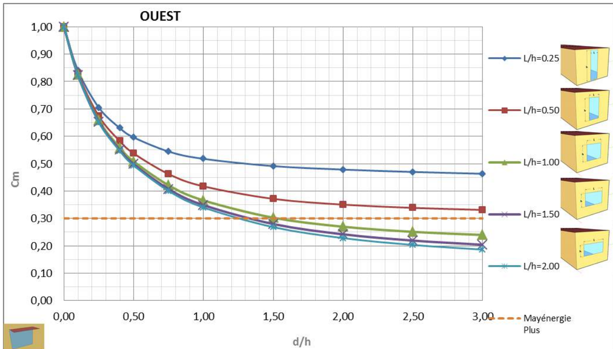
Figure 6-25 : Variations de C_m en fonction de la profondeur du débord, pour différentes fenêtres orientées Ouest
