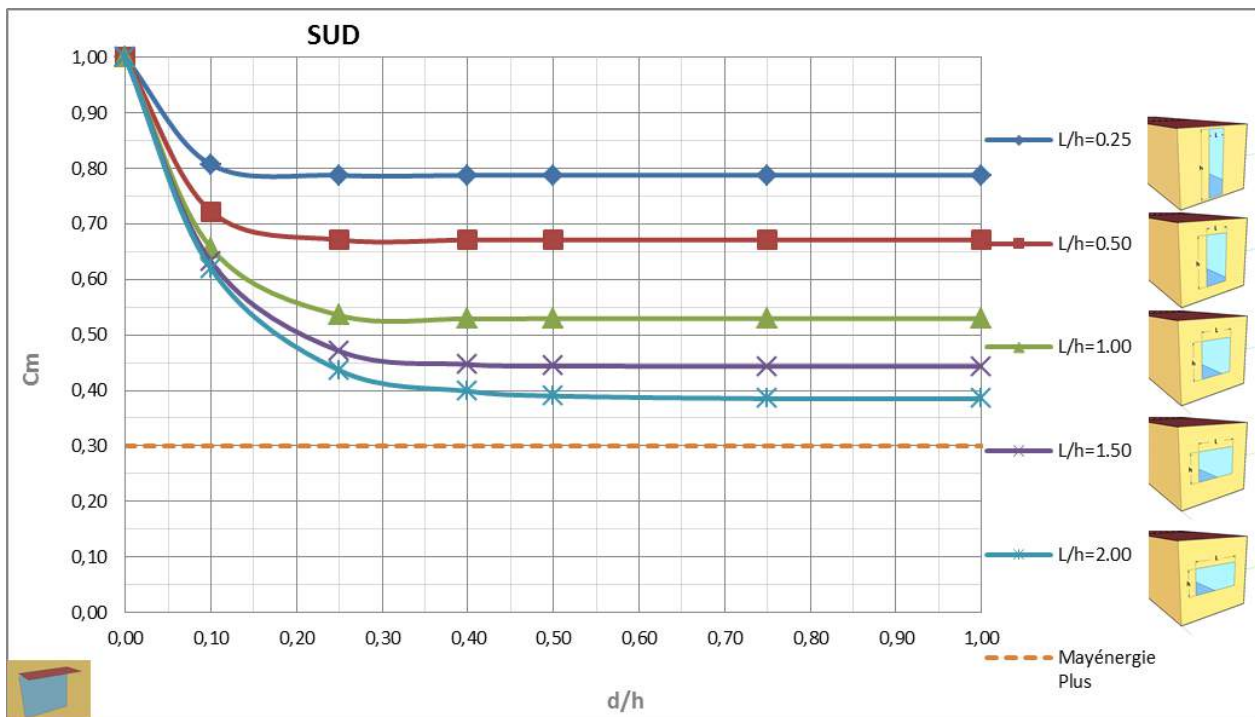
Figure 6-23 : Variations de C_m en fonction de la profondeur du débord, pour différentes fenêtres orientées Sud
