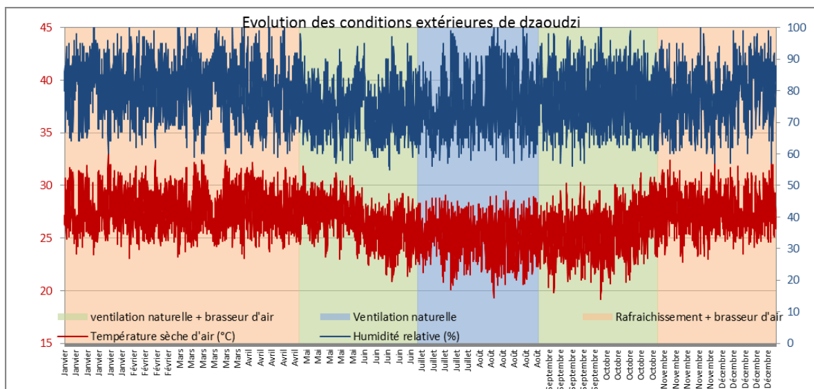
Figure 4.1 Exemple de scénarios d'utilisation des options de rafraîchissement en fonction de la température du local
