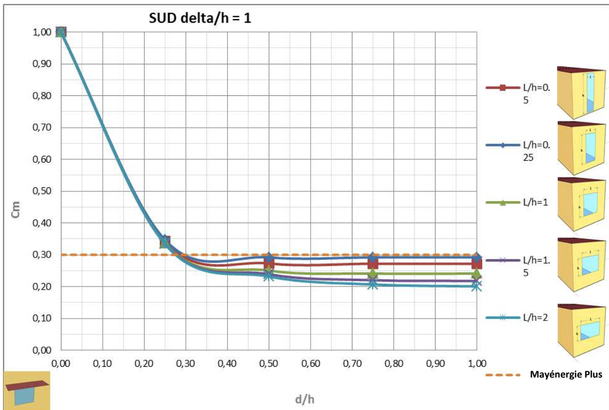
Figure 6-33 : Valeurs de C_m en fonction de la profondeur du débord pour une extension de débord \delta/h = 1 , pour des fenêtres orientées Sud
