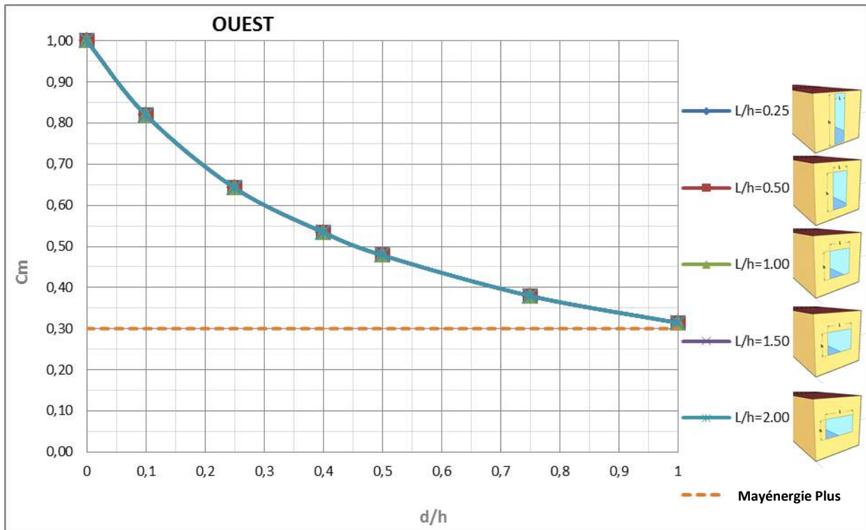
Figure 6-38 : Valeurs de C_m en fonction de la profondeur du débord pour différentes fenêtres orientées Ouest
