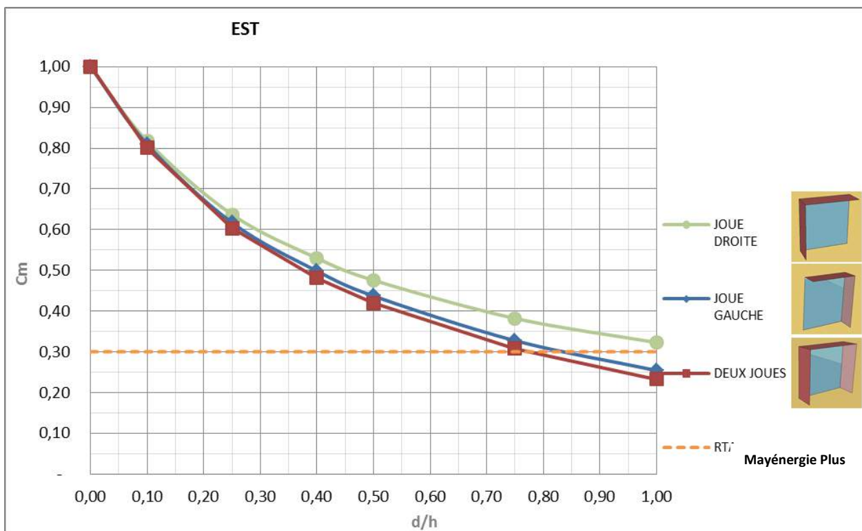
Figure 6-41 : Valeurs de Cm en fonction de la profondeur du débord, pour une fenêtre carrée, orientée Est
