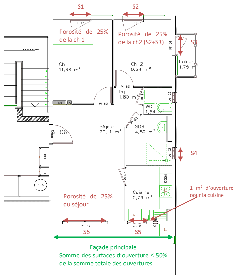
Figure 3.1 : Ventilation d'un logement sur trois façades
