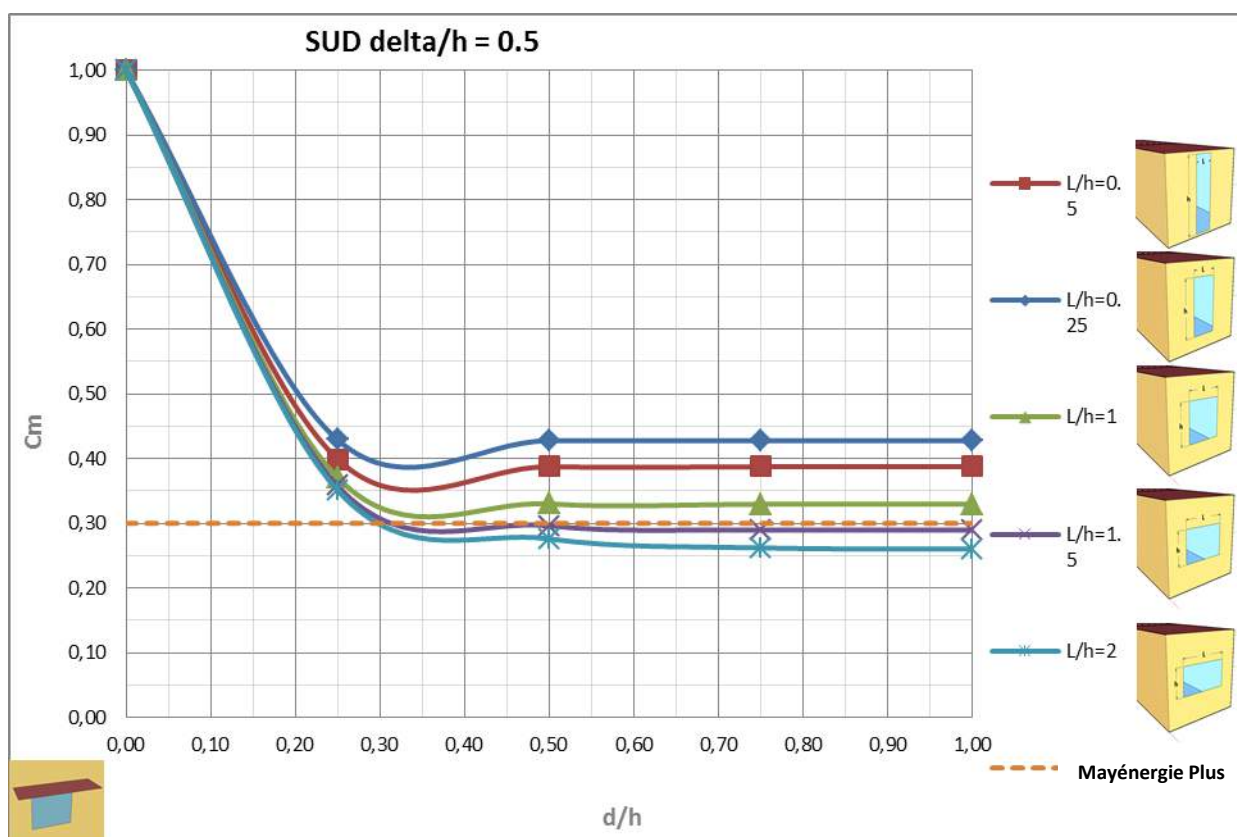
Figure 6-31 : Valeurs de C_m en fonction de la profondeur du débord pour une extension de débord \delta/h = 0.50 , pour des fenêtres orientées Sud
