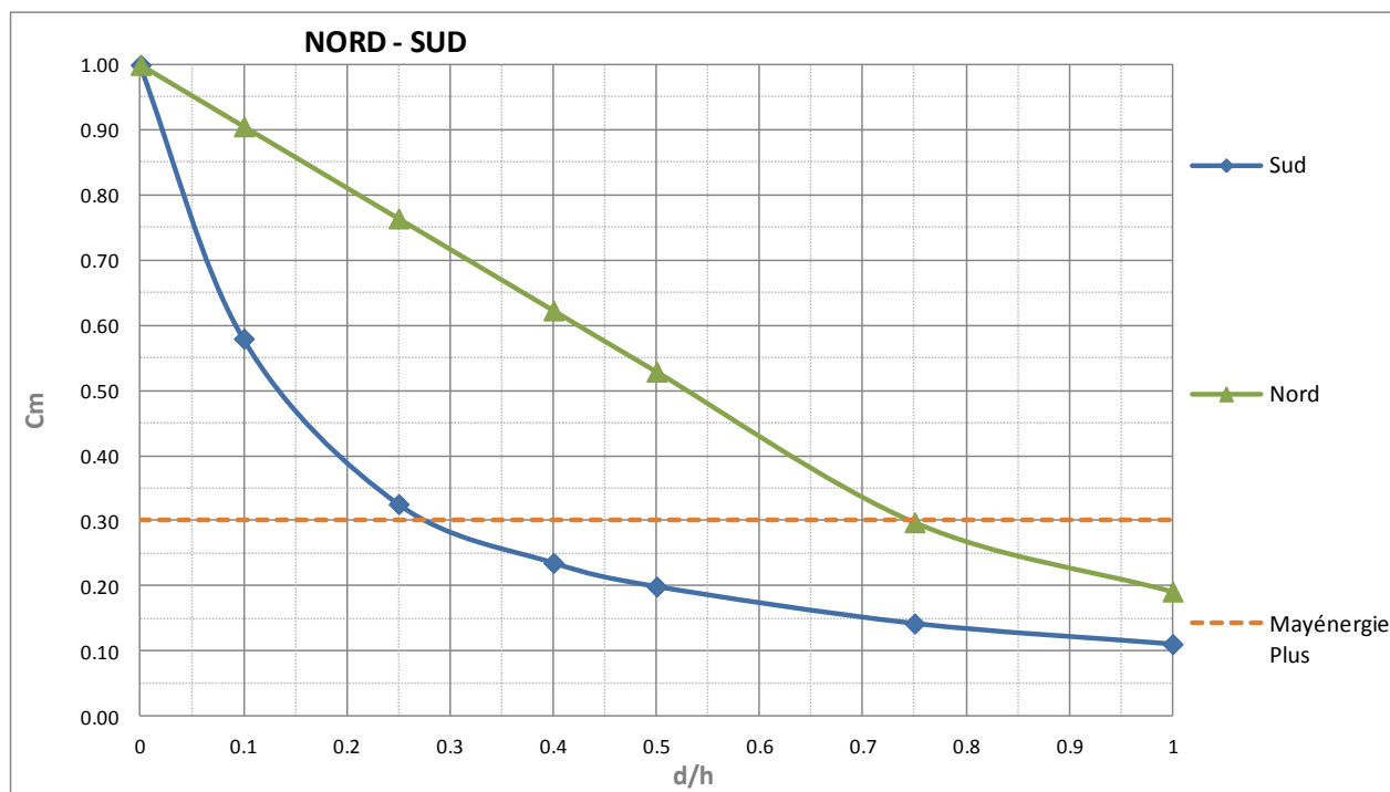
Figure 6-12 : Variation de C_m en fonction de la profondeur du débord pour des parois opaques verticales (murs) orientées nord ou sud
