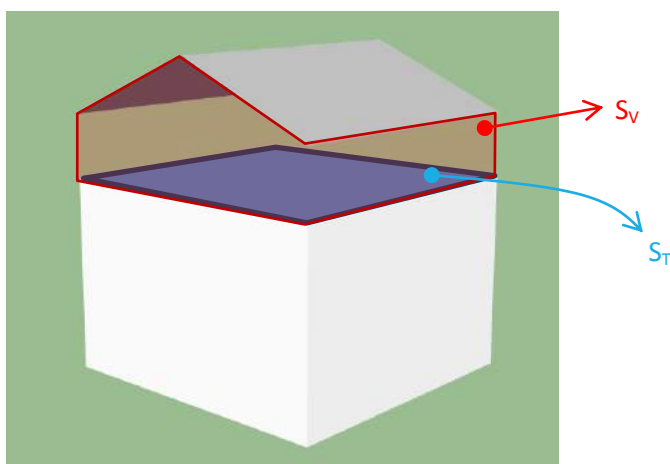
Figure 6-9 Définition d'un pare-soleil ventilé (ou sur-toiture)
