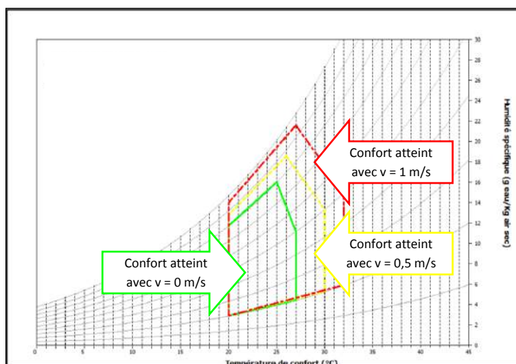
Figure 6-7 : Les trois zones de confort de Givoni pour une vêtue légère (pantalon et chemise manches courtes) et une activité de type bureau. Lorsque la vitesse d'air intérieur est égale à 1 m/s, les conditions de confort sont délimitées par le polygone rouge (jusqu'à 32°C en termes de température et jusqu'à 95% en termes d'humidité).
