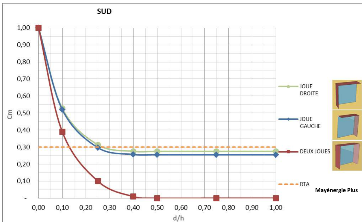
Figure 6-40 : Valeurs de C_m en fonction de la profondeur du débord, pour une fenêtre carrée, orientée Sud
