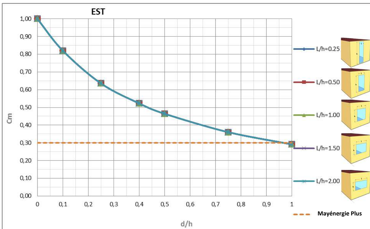
Figure 6-37 : Valeurs de C_m en fonction de la profondeur du débord, pour différentes fenêtres orientées Est
