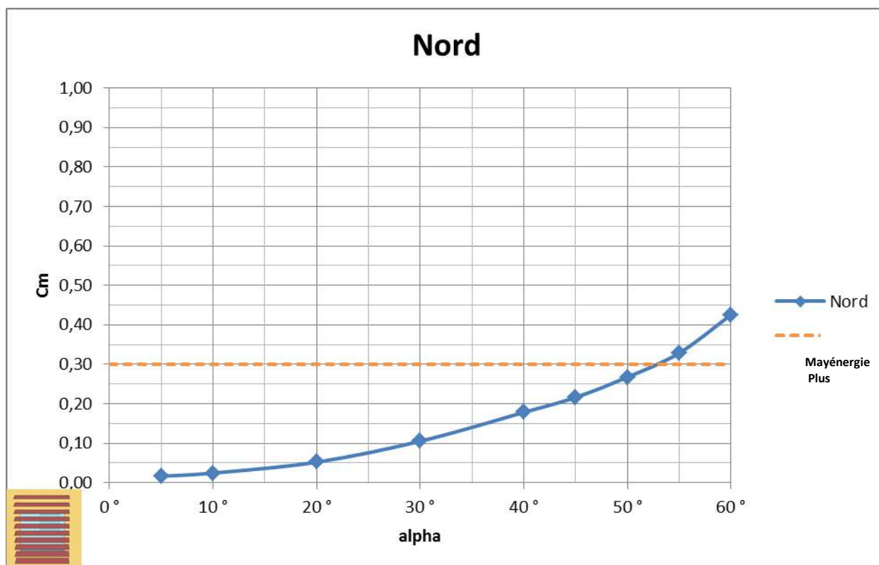
Figure 6-45 : Valeurs de Cm en fonction de l'orientation des lames pour une fenêtre carrée, orientée Nord
