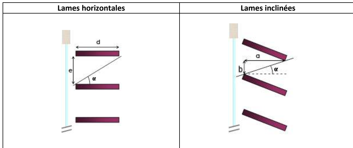
Figure 6-43 Définition de l'angle \alpha pour des lames horizontales et inclinées
