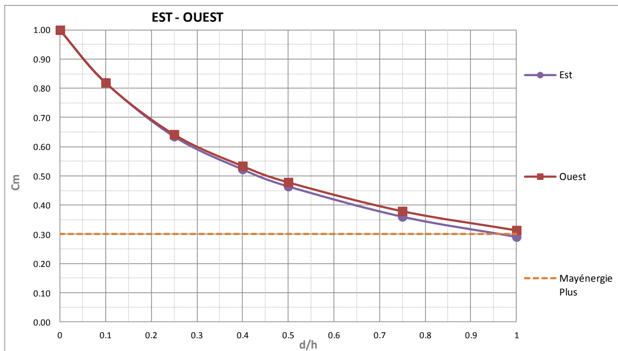
Figure 6-13 : Variation de C_m en fonction de la profondeur du débord pour des parois opaques verticales (murs) orientées est ou ouest
