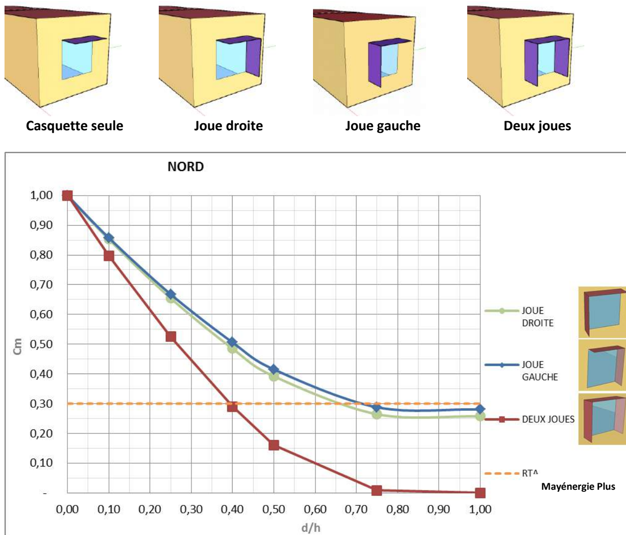
Figure 6-39 : Valeurs de C_m en fonction de la profondeur du débord, pour une fenêtre carrée, orientée Nord
