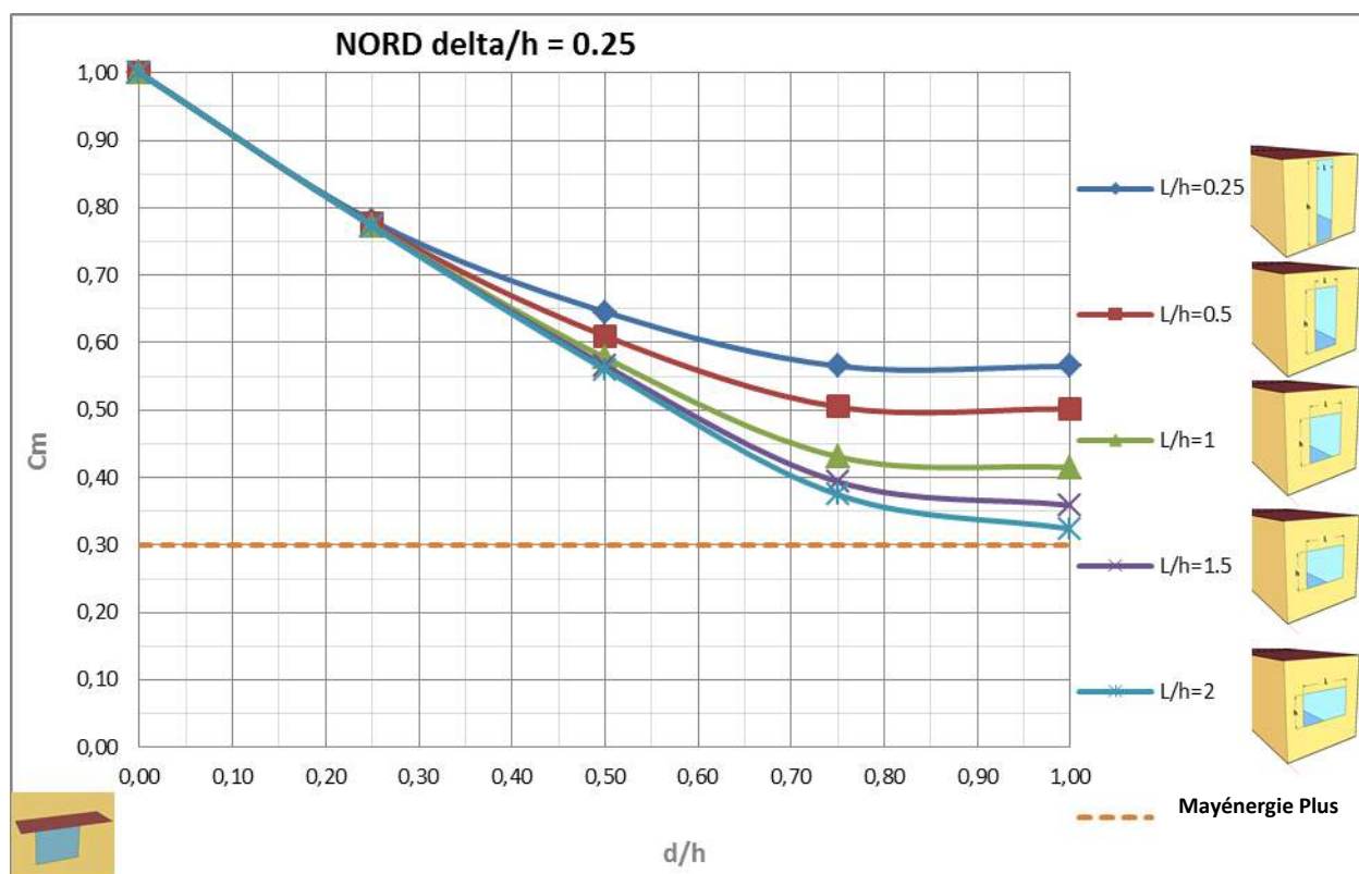
Figure 6-26 : Valeurs de C_m en fonction de la profondeur du débord pour une extension de débord \delta/h = 0.25 , pour des différentes fenêtres orientées Nord
