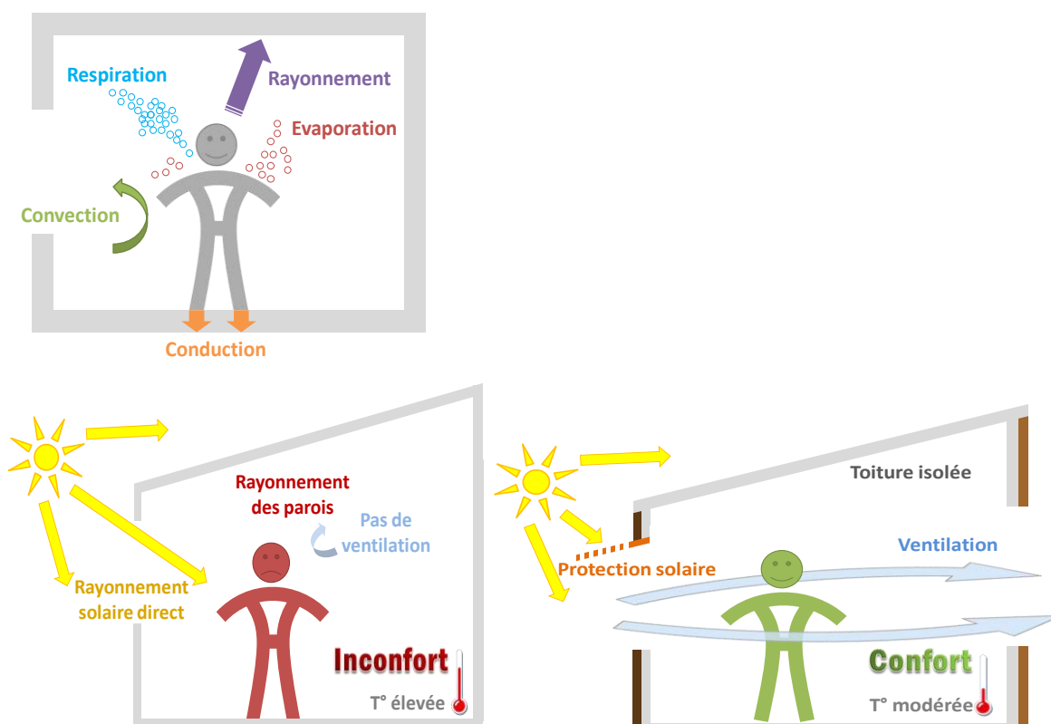
Figure 6-6 : Les conditions de confort (protection solaire et ventilation naturelle traversante (figure de droite). La création d'une vitesse d'air de 1m/s sur l'occupant permet de baisser la température ressentie de 4°C par rapport à la température d'air (figure de gauche).
