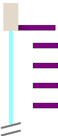
Figure 6-44 Cas où les lames sont déportées de la façade à protéger
