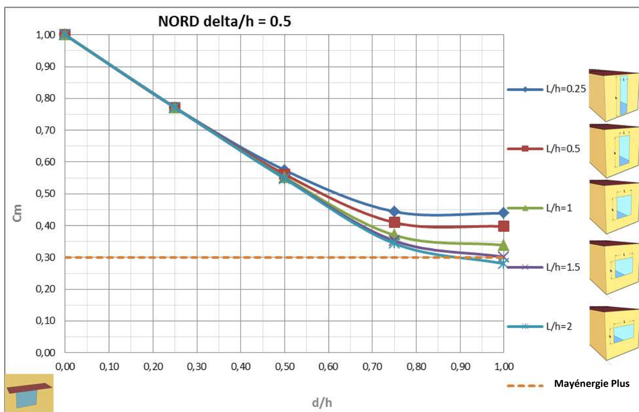
Figure 6-27 : Valeurs de C_m en fonction de la profondeur du débord pour une extension de débord \delta/h = 0.5 , pour différentes fenêtres orientées Nord
