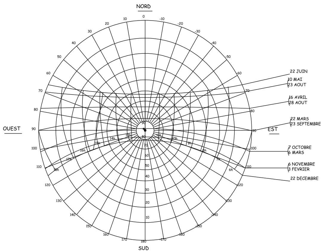
Figure 6-4 : Diagramme solaire de Mayotte. Attention, ce diagramme n'est utilisable que pour l'île de Mayotte.
