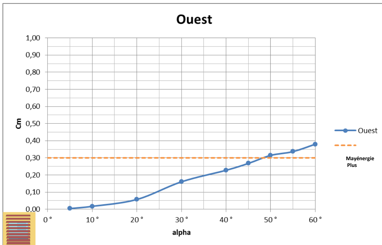
Figure 6-48 : Valeurs de Cm en fonction de l'orientation des lames pour une fenêtre carrée, orientée Ouest
