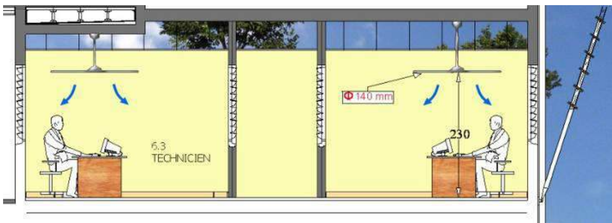
Figure 3.3 : Installation de brasseurs d'air dans des bureaux.
