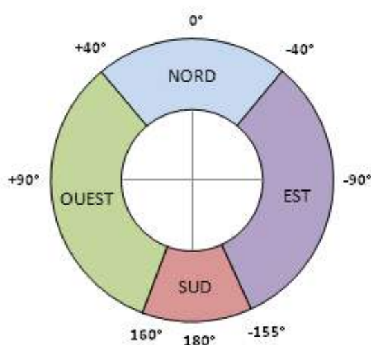
Figure 6-11 : Définition des orientations des baies et parois opaques en fonction de l'azimut
