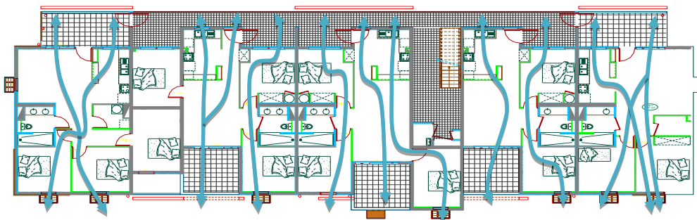
Figure 3.2 : Ventilation à l'échelle du bâtiment en logements collectifs
