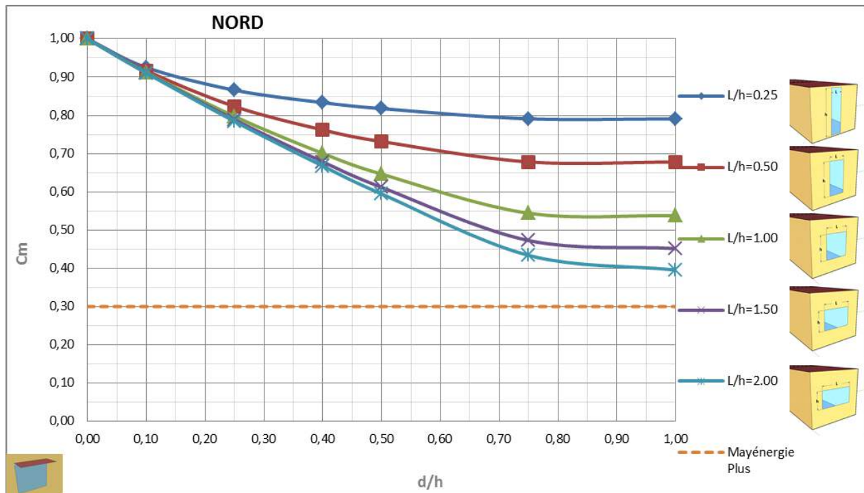
Figure 6-22 : Variations de C_m en fonction de la profondeur du débord, pour différentes fenêtres orientées Nord
