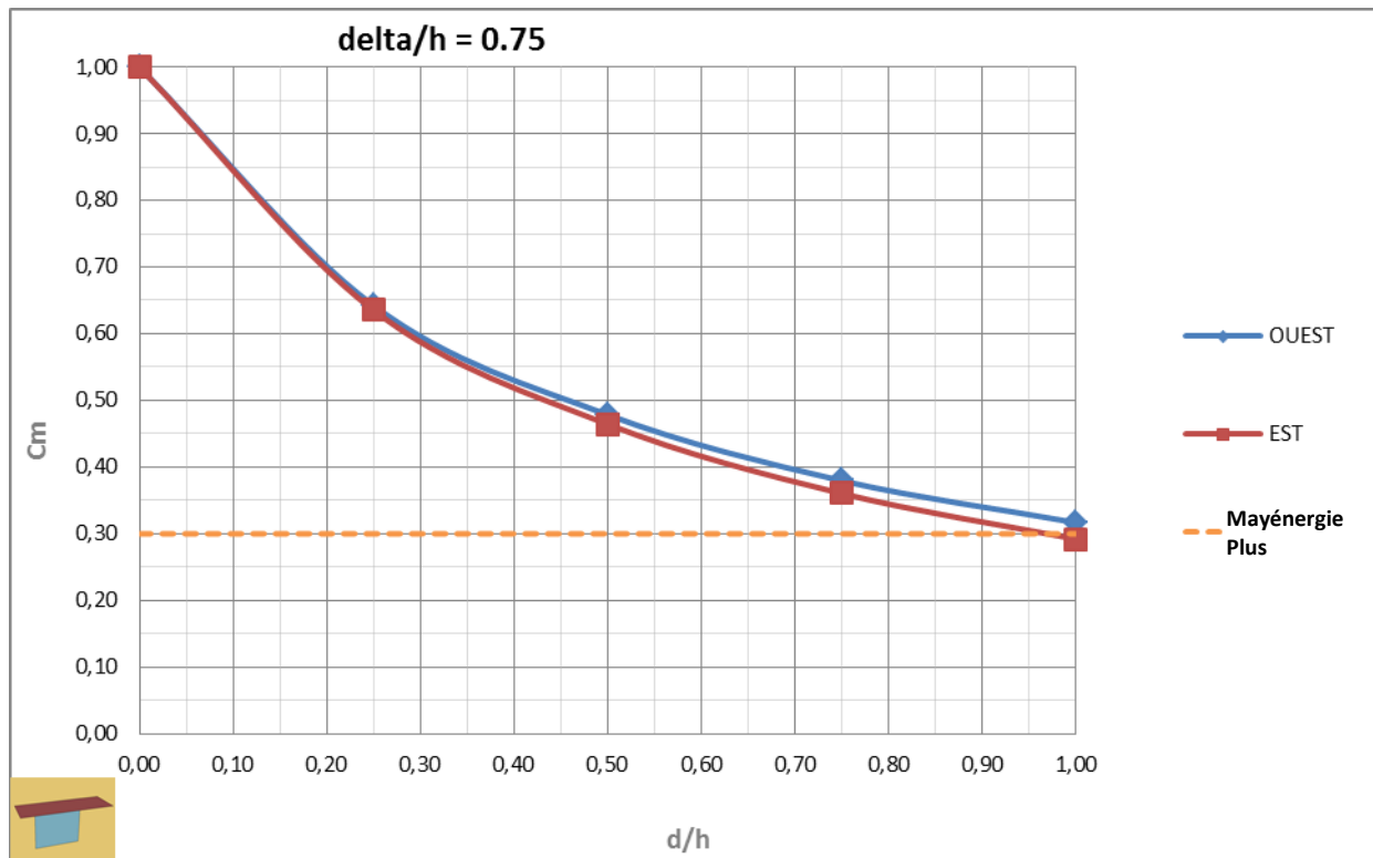
Figure 6-34 : Valeurs de C_m en fonction de la profondeur du débord, pour des fenêtres carrées, orientées Est et Ouest
