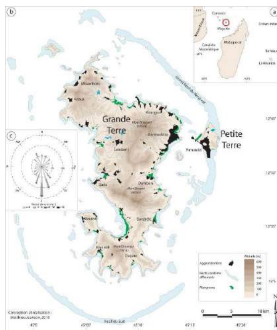
Figure 6-1 : cartographie des régimes de vent à Mayotte
