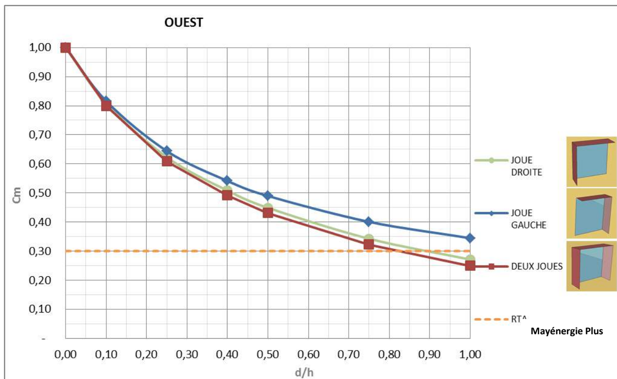
Figure 6-42 : Valeurs de Cm en fonction de la profondeur du débord, pour une fenêtre carrée, orientée Ouest
