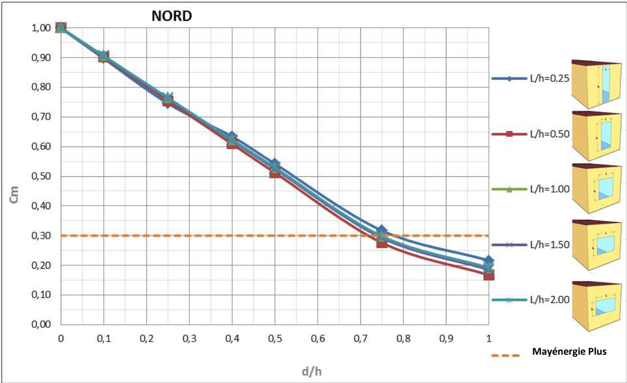
Figure 6-35 : Valeurs de Cm en fonction de la profondeur du débord, pour différentes fenêtres orientées Nord
