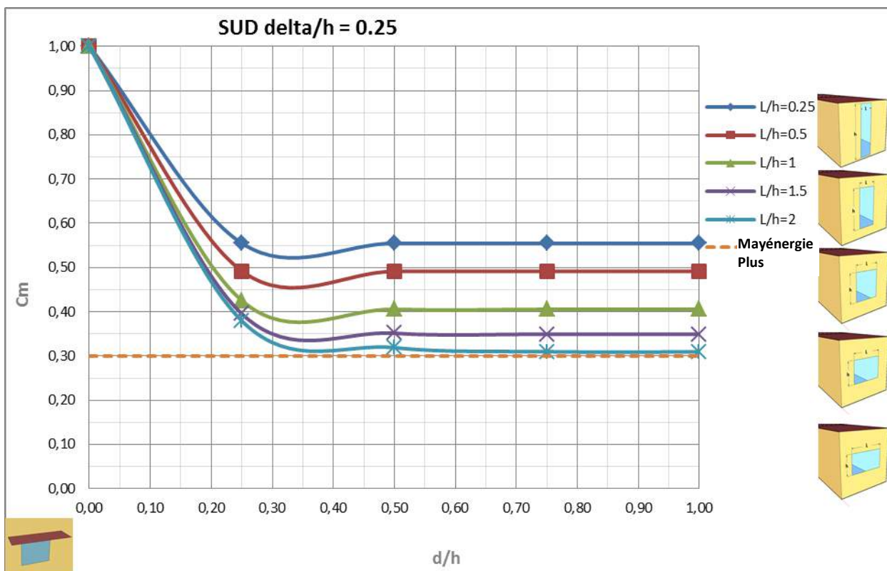
Figure 6-30 : Valeurs de C_m en fonction de la profondeur du débord pour une extension de débord \delta/h = 0.25 , pour des fenêtres orientées Sud
