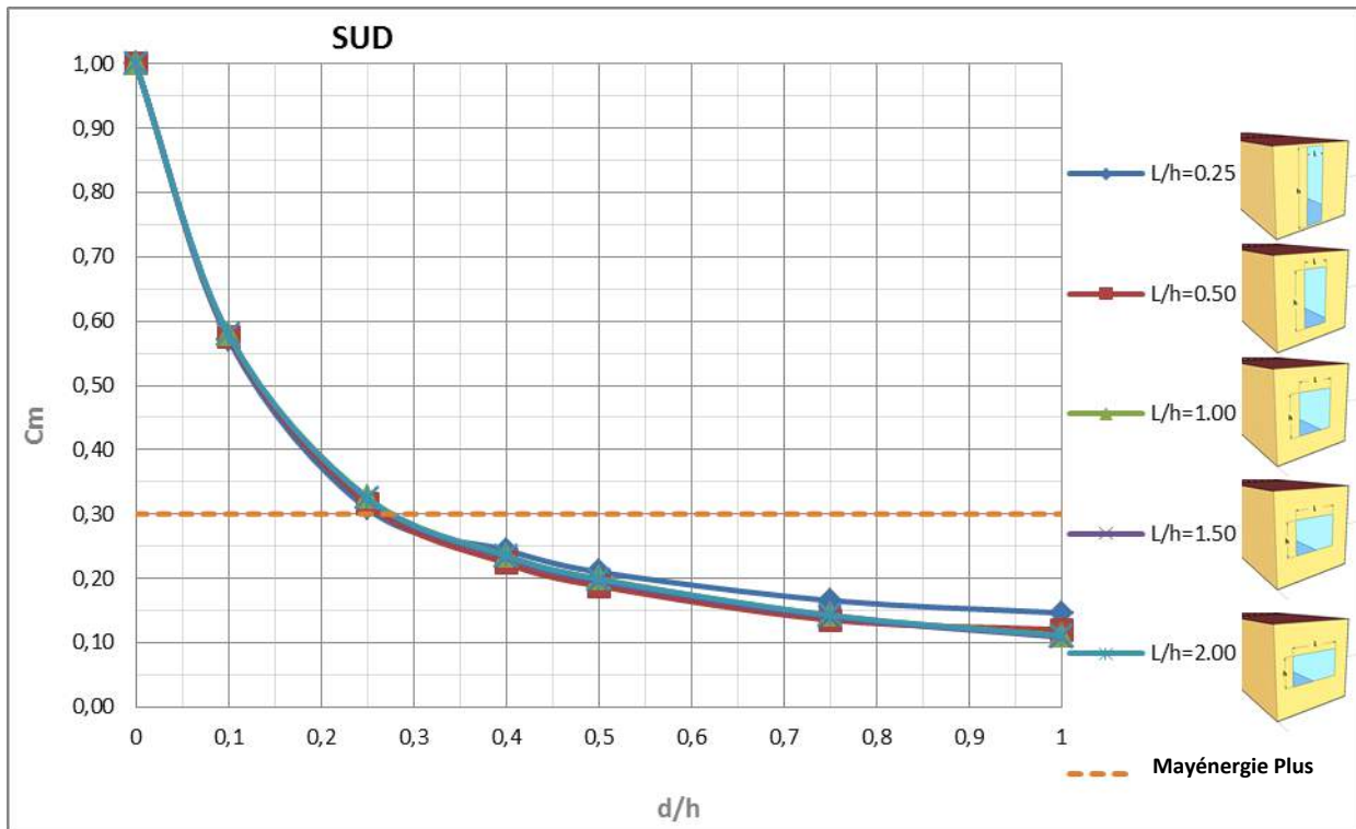
Figure 6-36 : Valeurs de C_m en fonction de la profondeur du débord, pour différentes fenêtres orientées Sud
