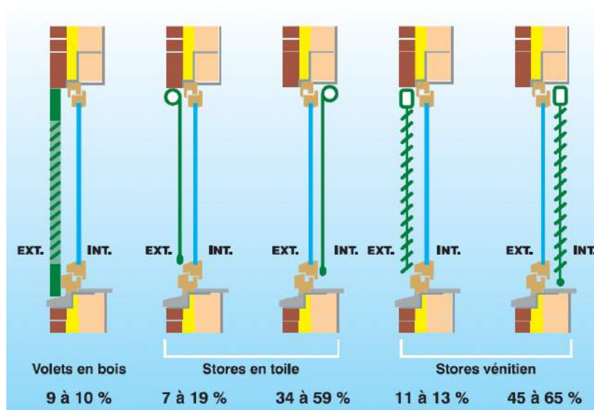
Figure 6-14 Facteurs solaires de différentes protections solaires pour un vitrage simple [Liébard 2005]
