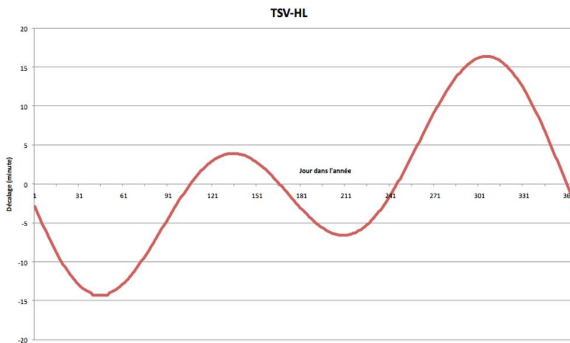
Figure 6-5 : Equation du temps pour Mayotte
