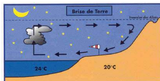
Figure 6-3 : Brise de terre Source atlas météo France
