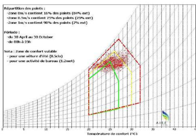
Figure 2.2 : Repr sentation du climat de Mayotte   l'aide des zones de confort de Givoni en saison humide (gauche) et en saison s che (droite).
