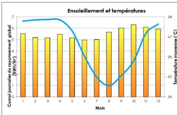
Figure 2.1 : Fiche climatique de la station de Pamandzi
