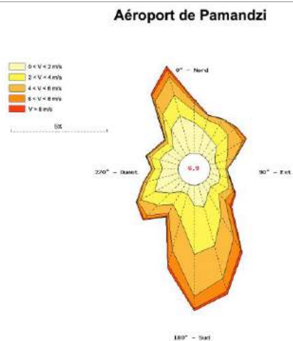
Figure 2.1 : Fiche climatique de la station de Pamandzi
