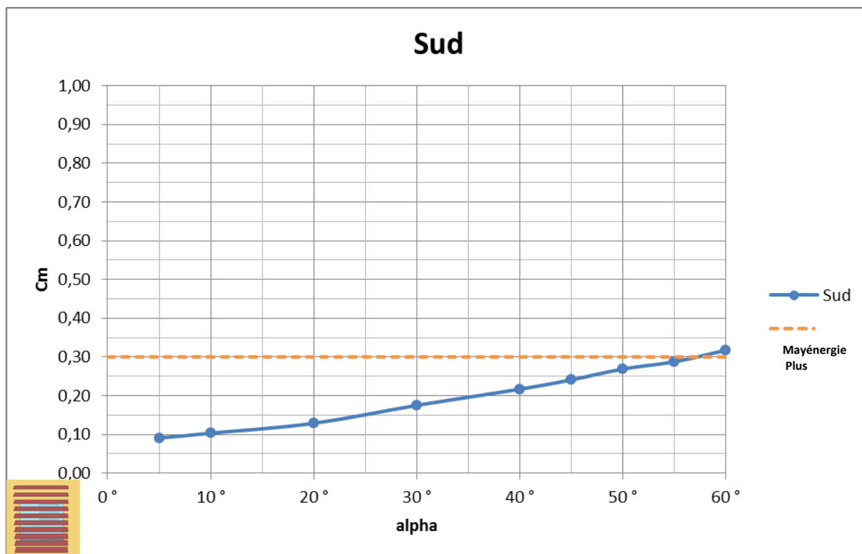
Figure 6-46 : Valeurs de Cm en fonction de l'orientation des lames pour une fenêtre carrée, orientée Sud
