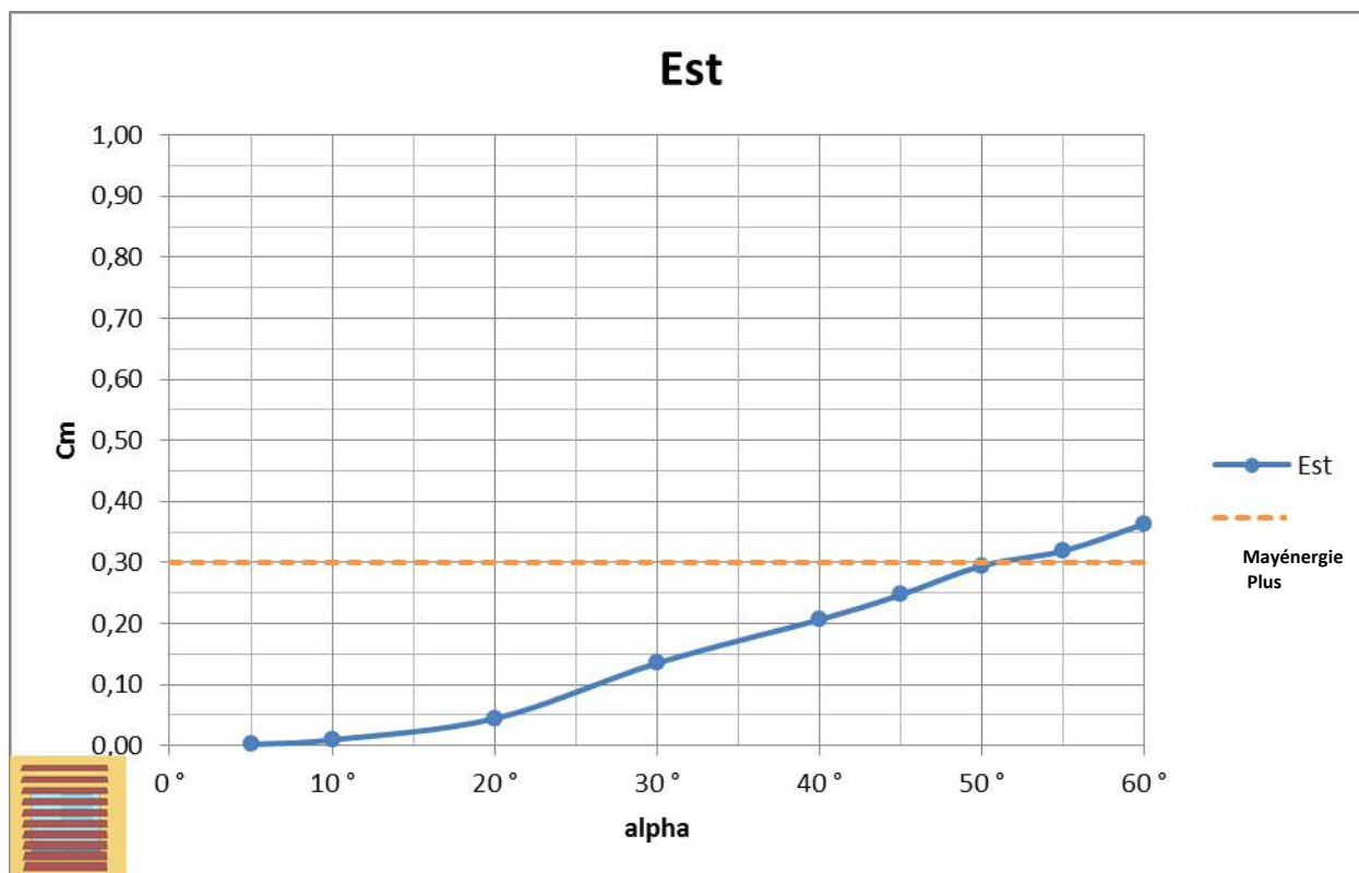
Figure 6-47 : Valeurs de Cm en fonction de l'orientation des lames pour une fenêtre carrée, orientée Est
