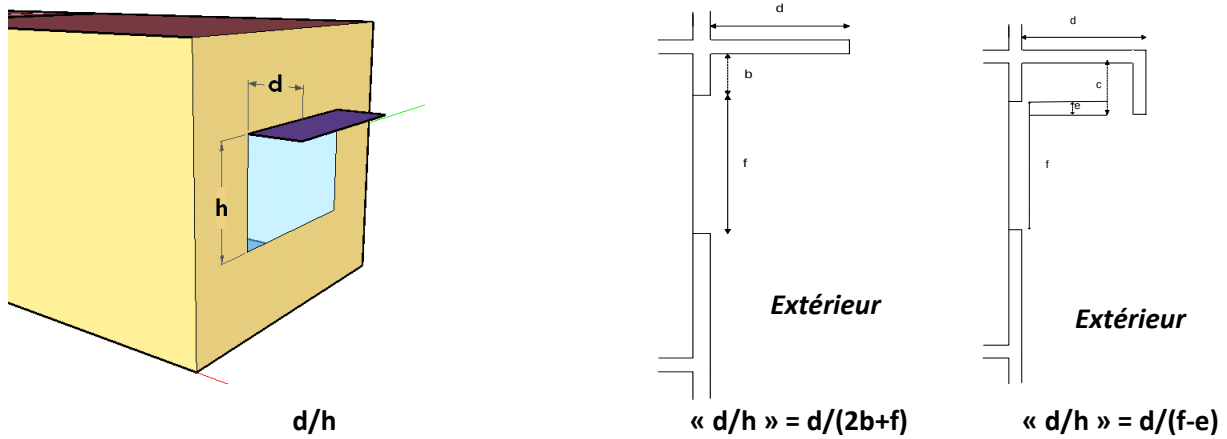
Figure 6-16: Définition du « d/h » équivalent
