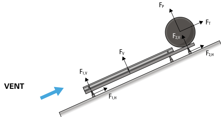
Figure 22 : Force de calcul des fixations basses ( F_1 ) et fixations hautes ( F_2 )
