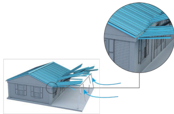
Figure 11 : Cas d'un auvent désolidarisé
